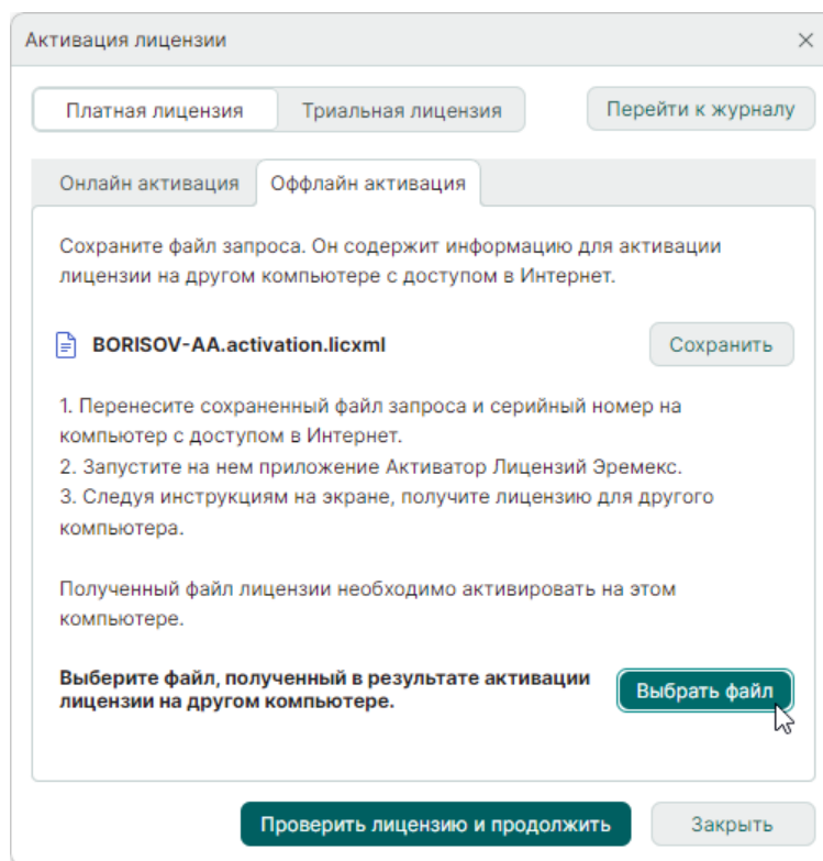
Рис. 50 Выбор файла лицензии
