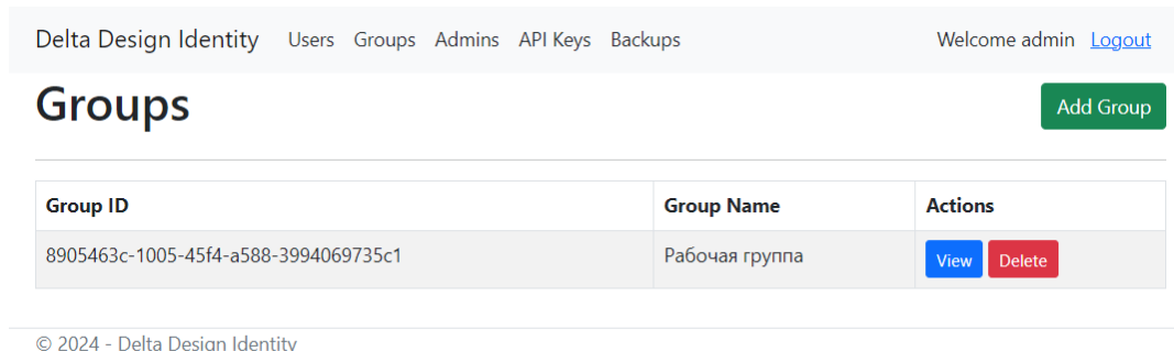
Рис. 72 Страница «Groups» (Группы)
