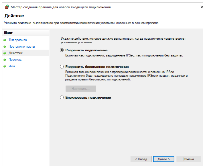
Рис. 60 Разрешите подключение, если выполнены указанные условия
