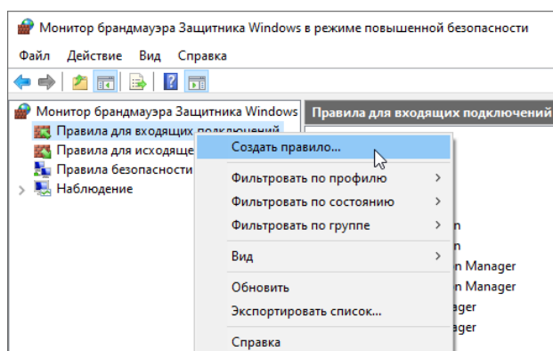
Рис. 57 Создание нового правила для работы брандмауэра
