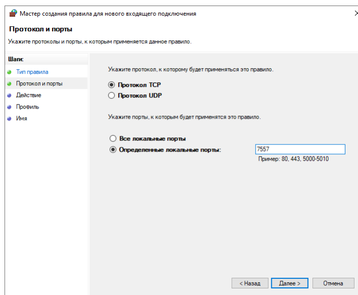
Рис. 59 Определение локального порта (7557)
