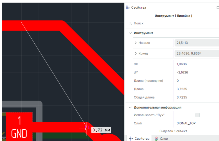
Рис. 93 Измерение расстояния
