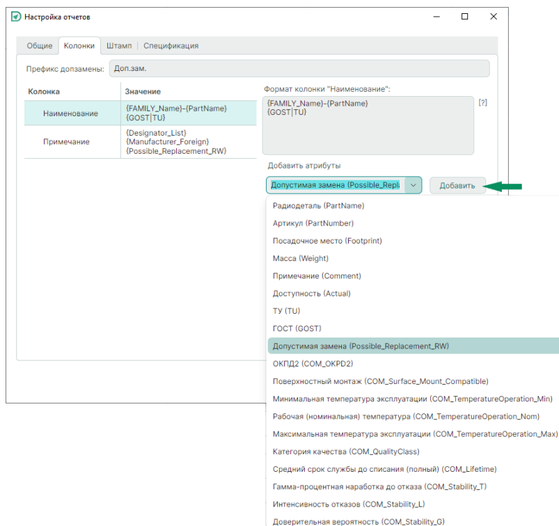
Рис. 24 Выбор атрибута для добавления в колонку
