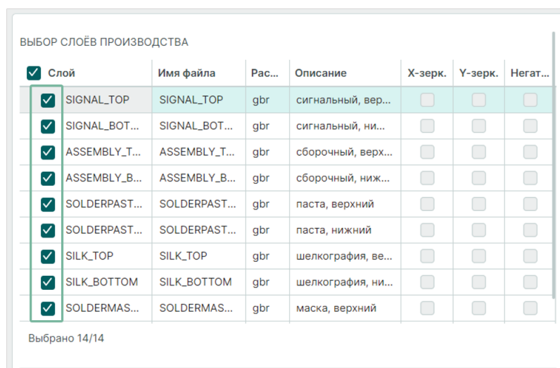
Рис. 137 Выбор слоев производства
