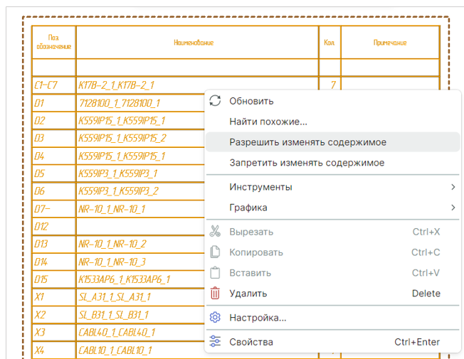
Рис. 111 Переход к изменению данных встроенного отчета
