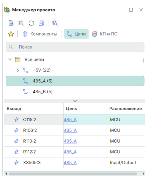
Рис. 488 Выводы компонентов, входящие в состав цепи
