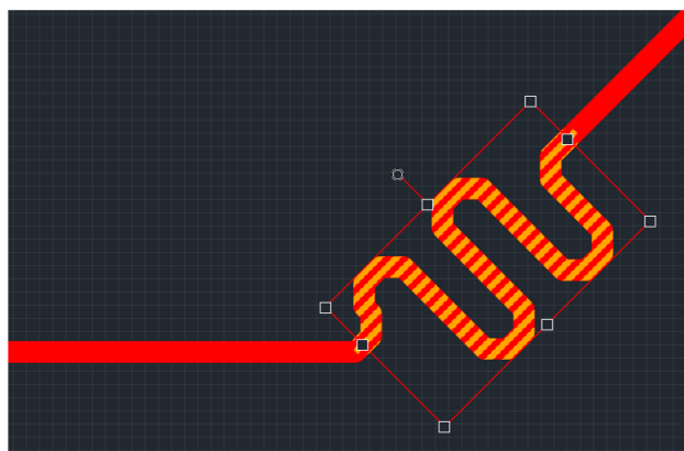
Рис. 275 Перемещение меандра по треку
