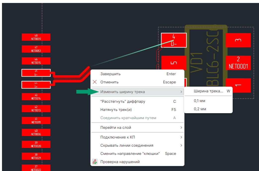
Рис. 341 Изменение ширины диффпары
