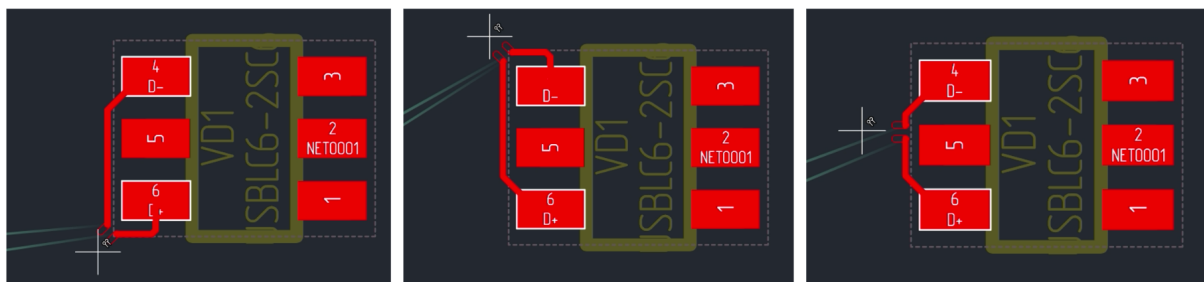
Рис. 330 Варианты несимметричного соединения с КП
