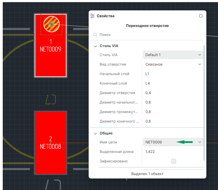
Рис. 185 Размещение ПО на КП без начала трассировки
