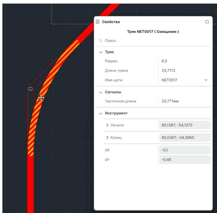
Рис. 292 Изменение скругления
