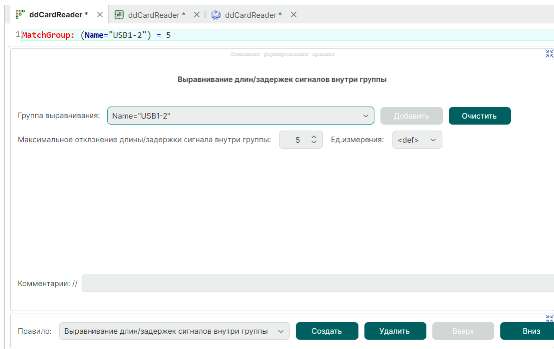
Рис. 370 Выравнивание длин/задержек сигналов внутри группы
