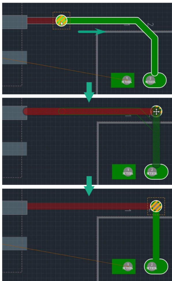
Рис. 270 Перемещение межслойного перехода с подключенными треками
