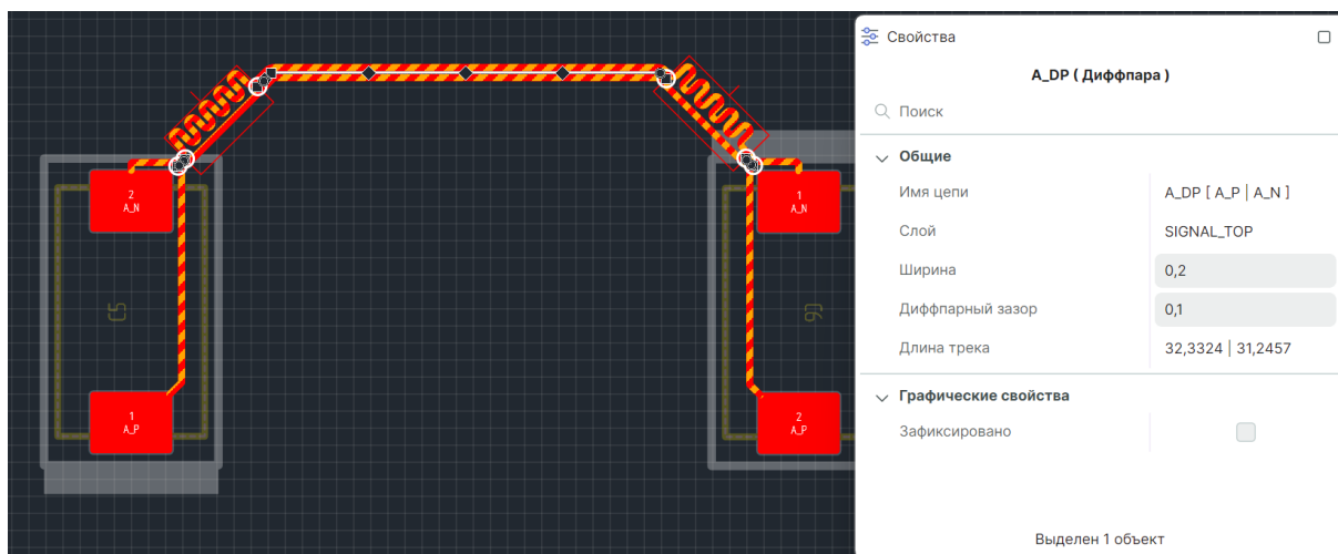
Рис. 351 Результат автоматического выравнивания дифференциальной пары
