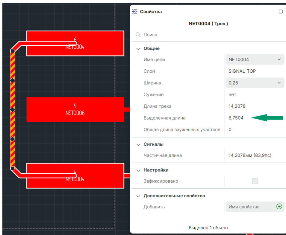
Рис. 201 Параметры трека - «Выделенная длина»
