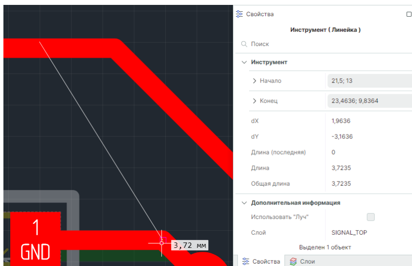
Рис. 93 Измерение расстояния
