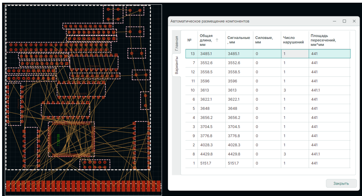
Рис. 148 Найденные варианты размещения компонентов
