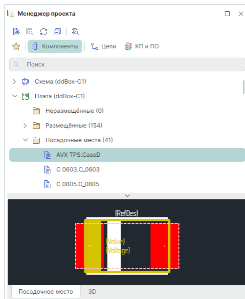
Рис. 157 Посадочные места в панели «Менеджер проекта»
