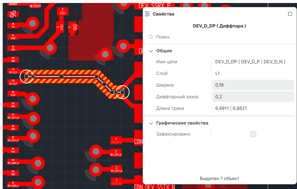
Рис. 324 Параметры диффпары
