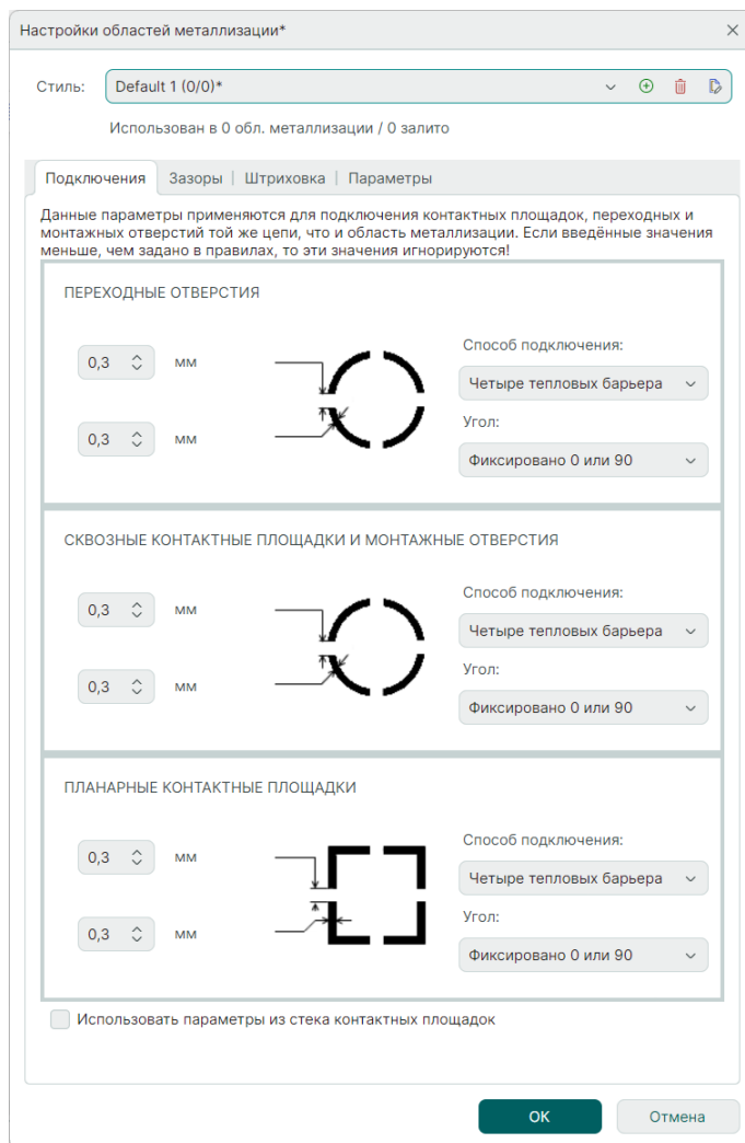
Рис. 443 Параметры термобарьеров по умолчанию
