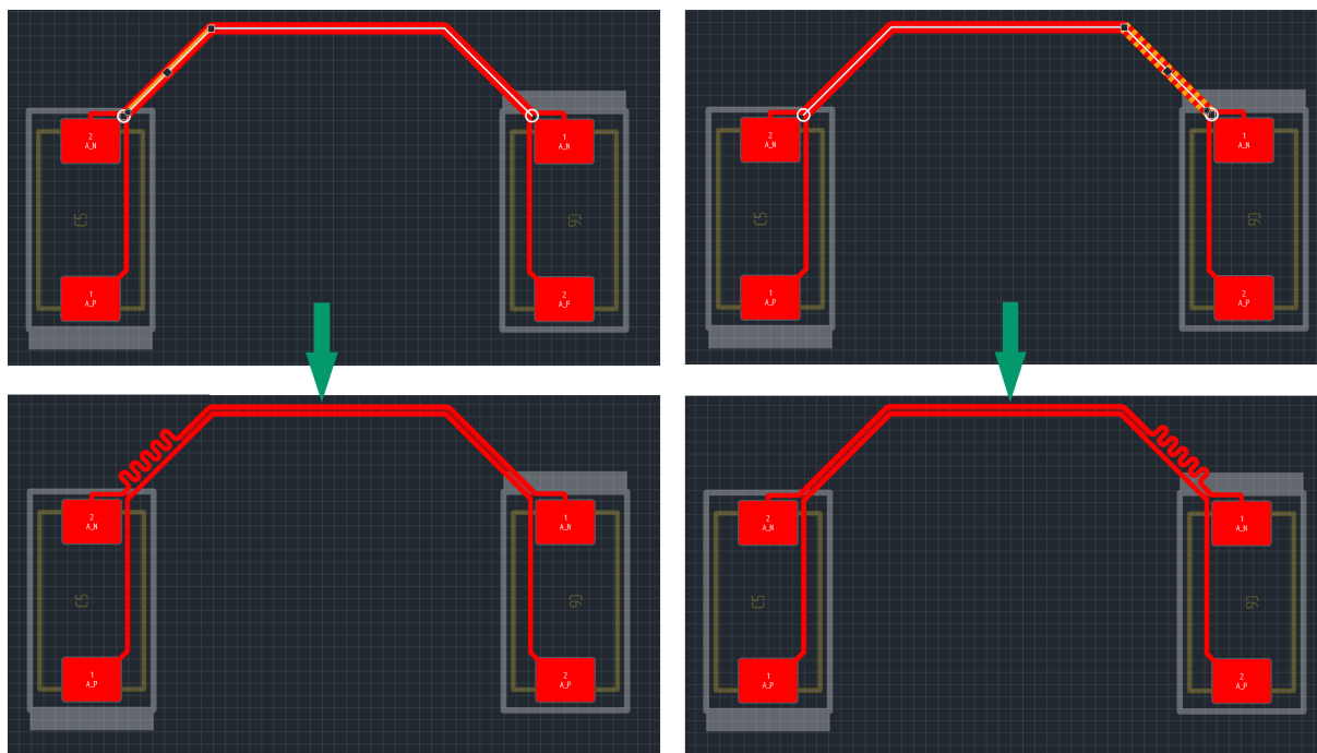
Рис. 352 Расположение меандра(ов) с учетом выделенного сегмента
