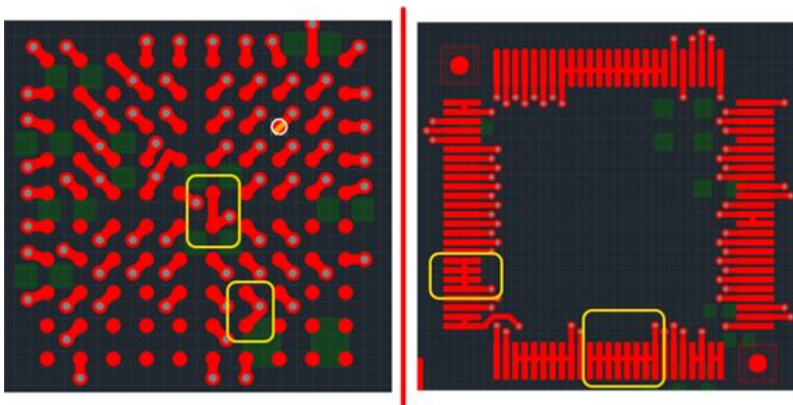
Рис. 316 Пример построения общих фанатов
