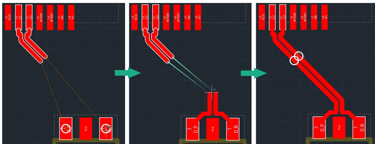
Рис. 346 Продолжение и завершение диффпары
