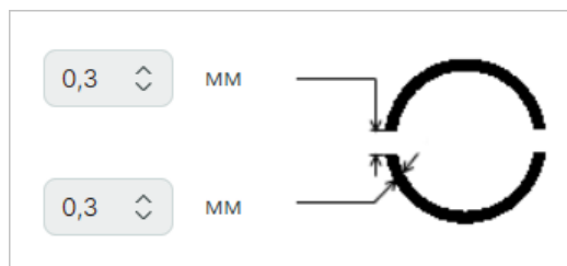
Рис. 446 Размеры термобарьера
