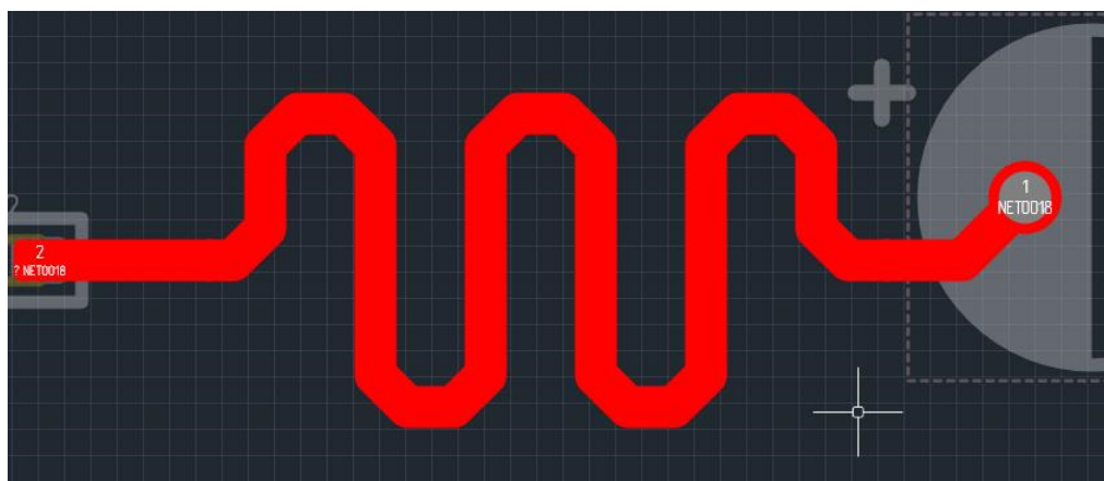
Рис. 272 Размещенный меандр
