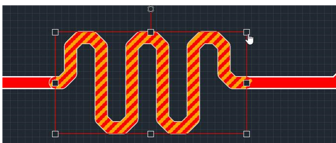
Рис. 276 Точки редактирования области размещения меандра
