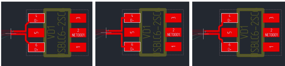
Рис. 329 Варианты симметричного соединения с КП
