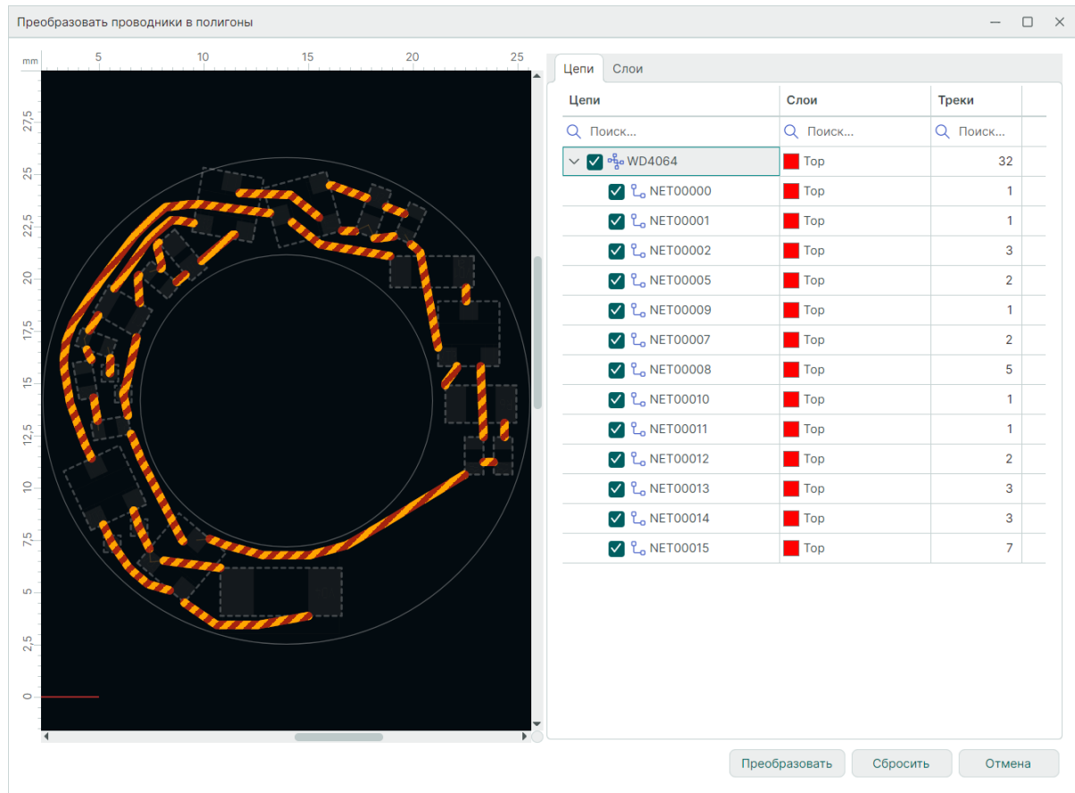
Рис. 403 Выбор проводников для преобразования в области металлизации
