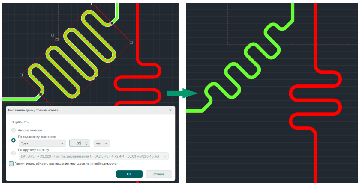
Рис. 392 Выравнивание длины трека/сигнала с уменьшением меандра
