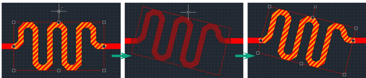
Рис. 278 Поворот меандра
