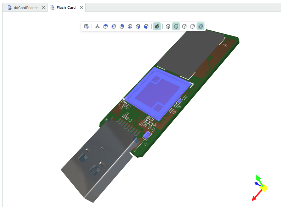
Рис. 540 Визуализация компонентов, к которым не привязана 3D модель
