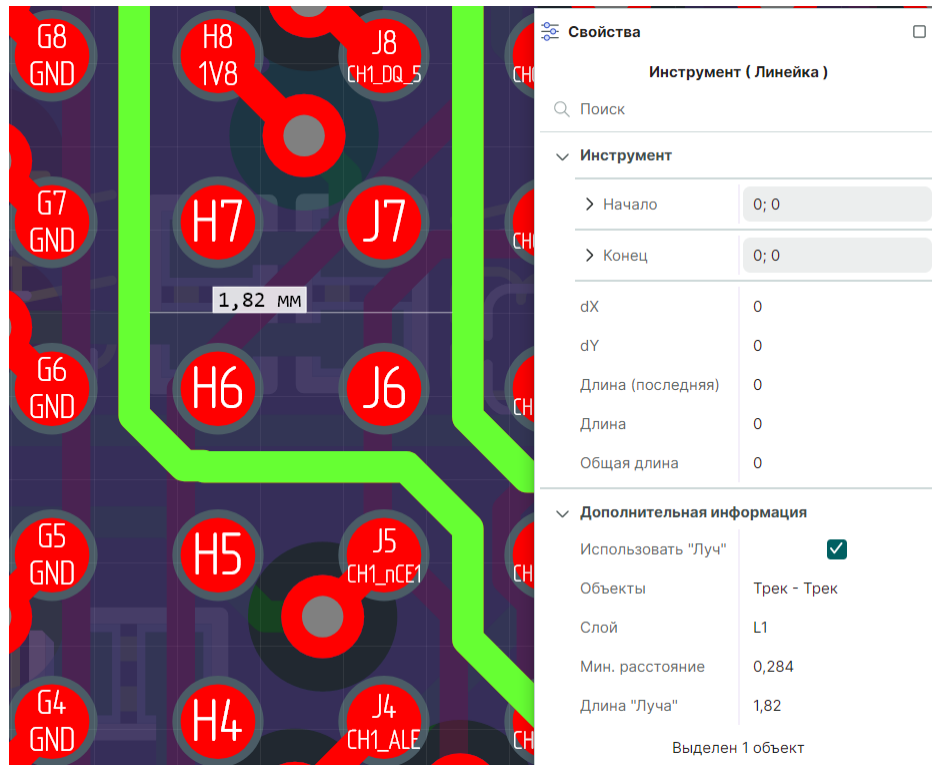
Рис. 94 Измерение расстояния с использованием «Луча»
