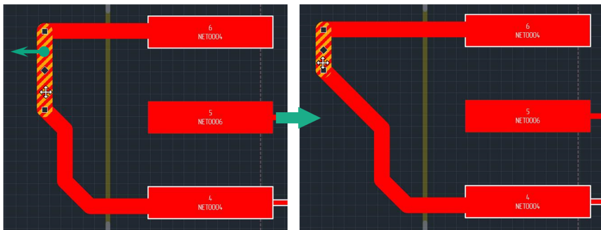
Рис. 258 Изменение соседствующих сегментов при перемещении
