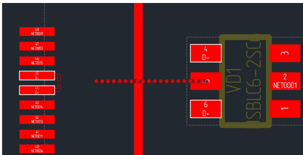
Рис. 333 Отображение некорректного варианта трассировки диффпары
