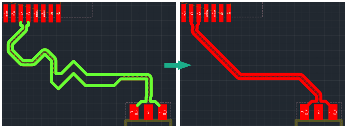
Рис. 348 Натяжение диффпары
