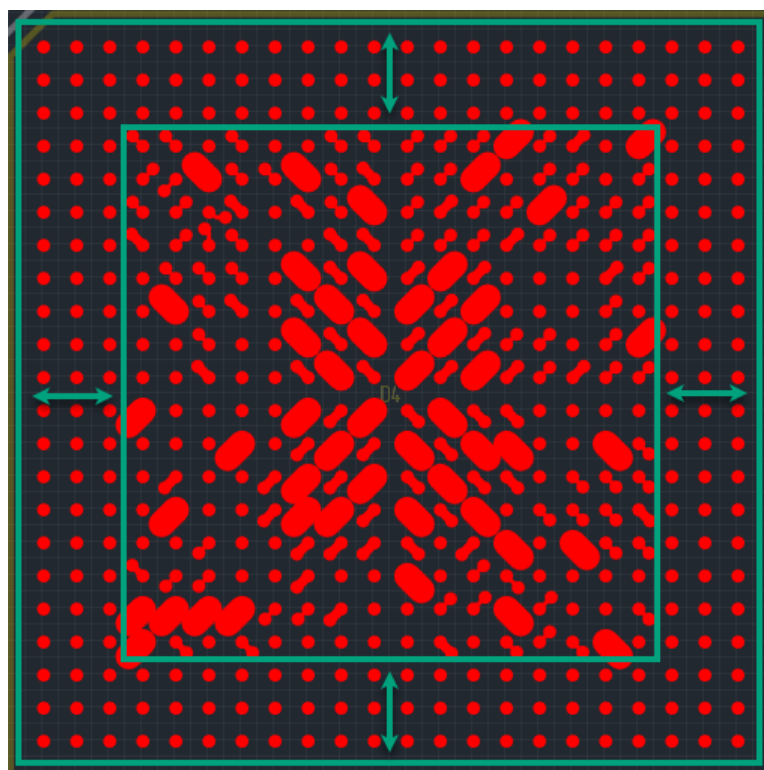
Рис. 298 Ряды и колонки матрицы BGA, для которых не построены фанавуты
