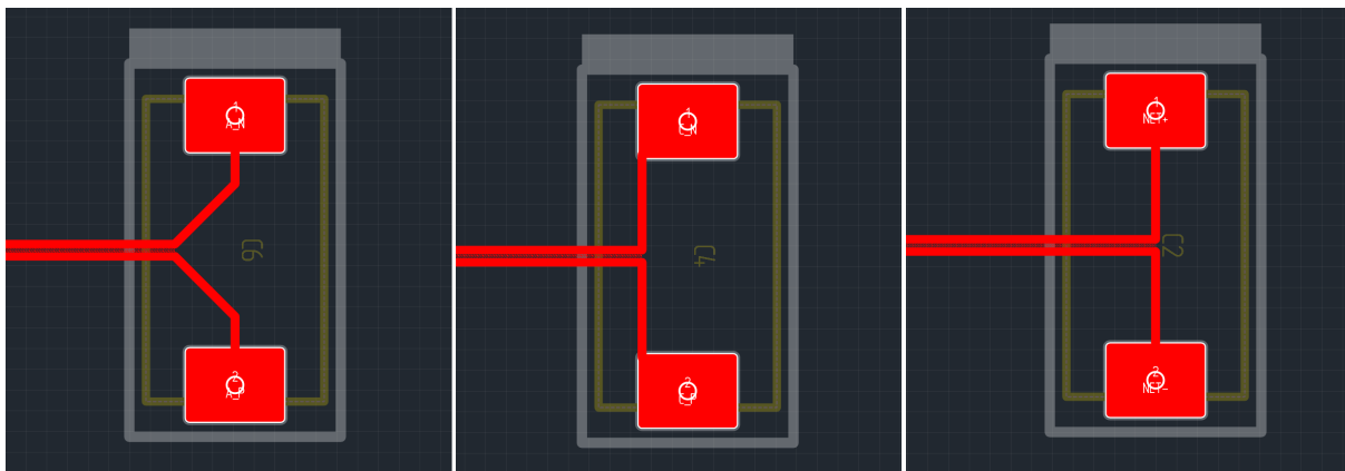
Рис. 339 Варианты симметричного завершения диффпары
