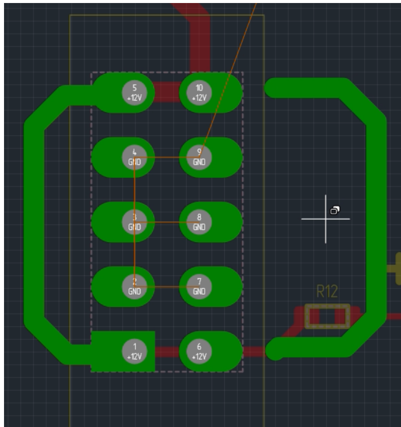
Рис. 421 Вращение копии трека при размещении
