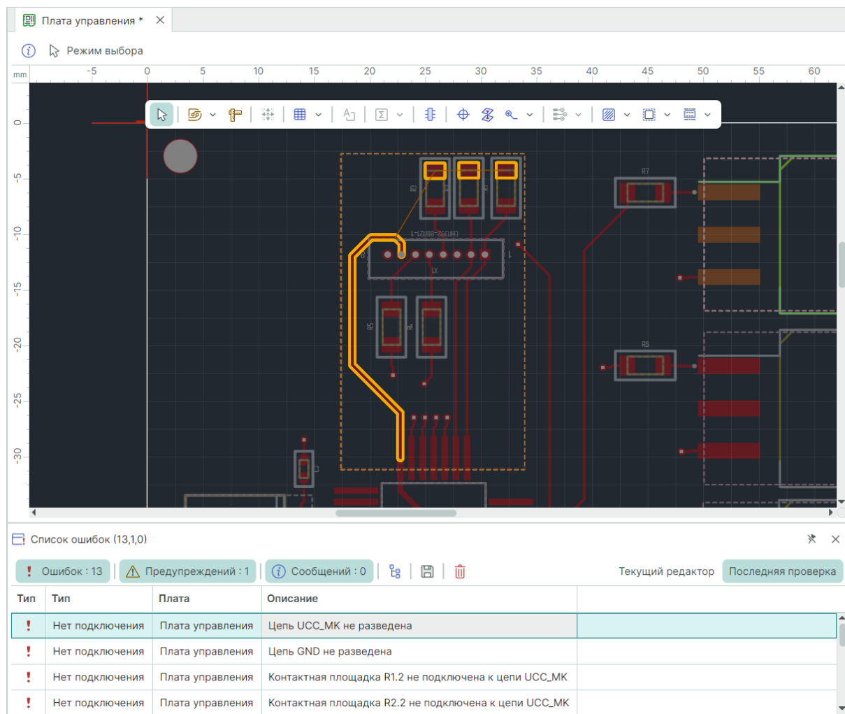
Рис. 535 Объекты, между которыми выявлено нарушение
