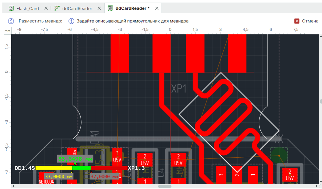
Рис. 379 Построение меандра на одном из сегментов трека
