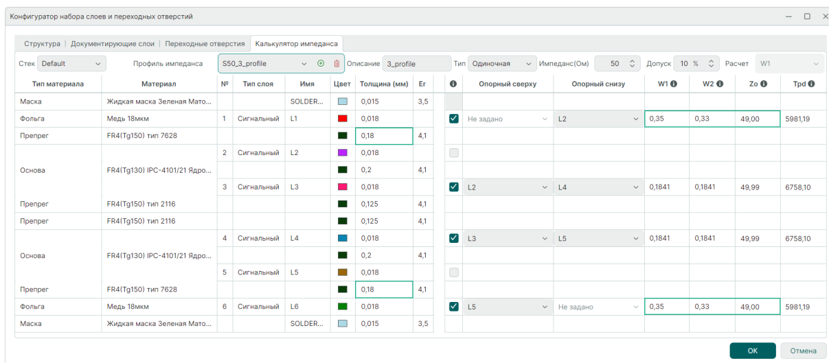
Рис. 50 Контроль рассчитанных параметров после изменения стека
