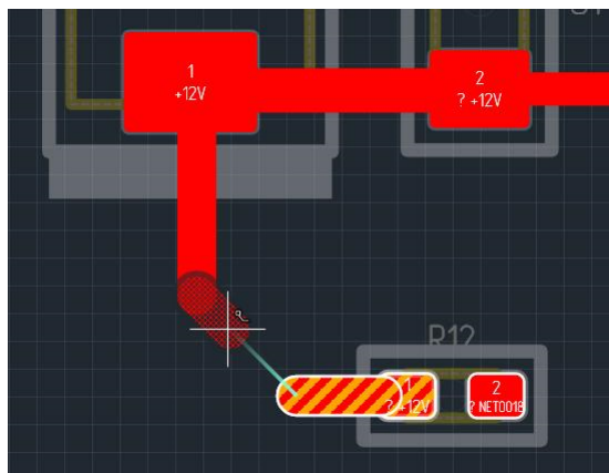
Рис. 256 Завершение трека с удаленными сегментами
