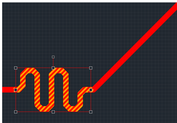
Рис. 274 Выделенный меандр на проводнике
