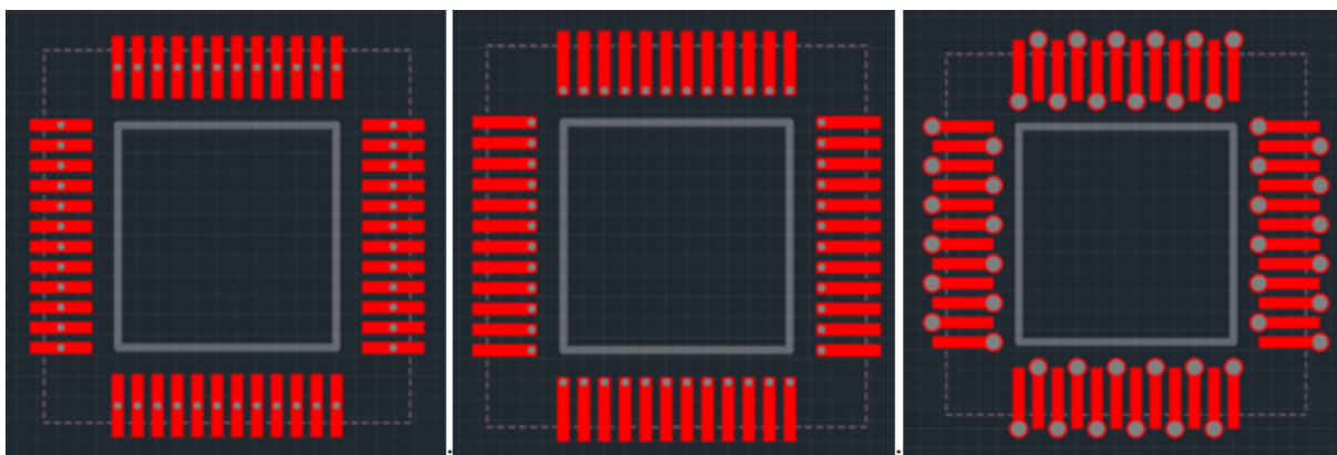
Рис. 311 Различные варианты расположения фанаутов относительно КП
