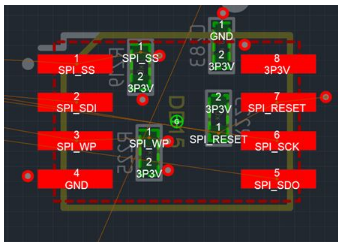
Рис. 198 Отображение номера контактной площадки и имени цепи
