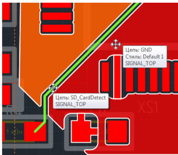
Рис. 456 Пример разделения области металлизации треком
