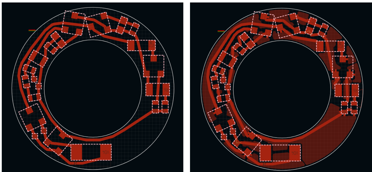
Рис. 404 Вид проводников до преобразования (слева) и после преобразования (справа) в области металлизации
