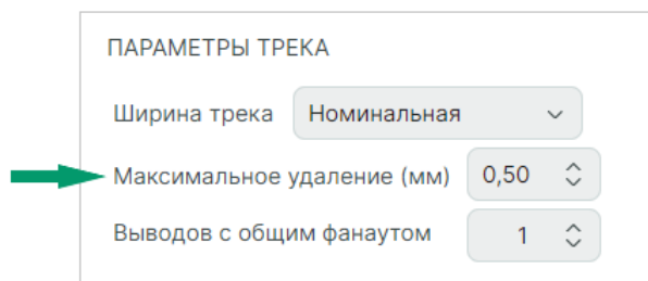
Рис. 314 Установка максимального расстояния между центром КП и центром ПО в фанaute
