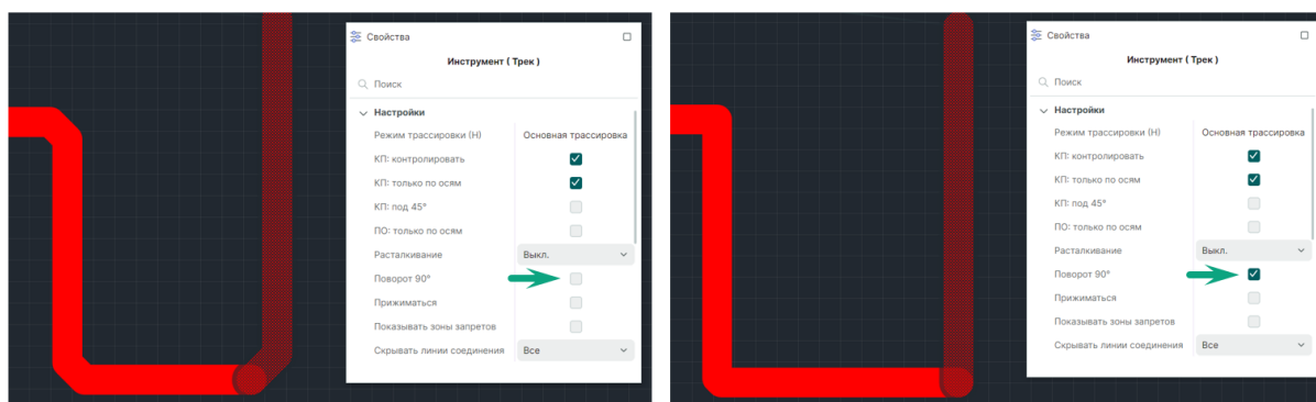
Рис. 235 Размещение трека с запретом и разрешением на трассировку под 90°
