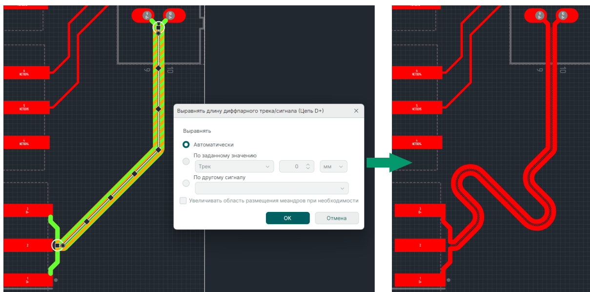
Рис. 391 Выравнивание дифференциальных пар
