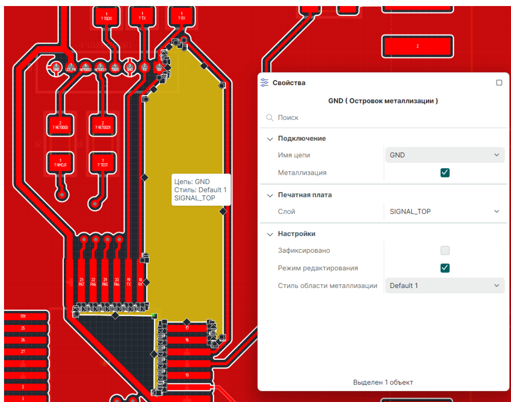
Рис. 463 Измененная геометрия островка металлизации
