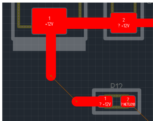
Рис. 254 Линия соединения после удаления сегмента трека
