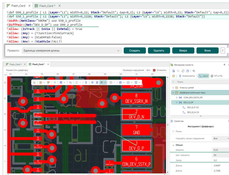
Рис. 53 Пример применения рассчитанных параметров к дифференциальной паре
