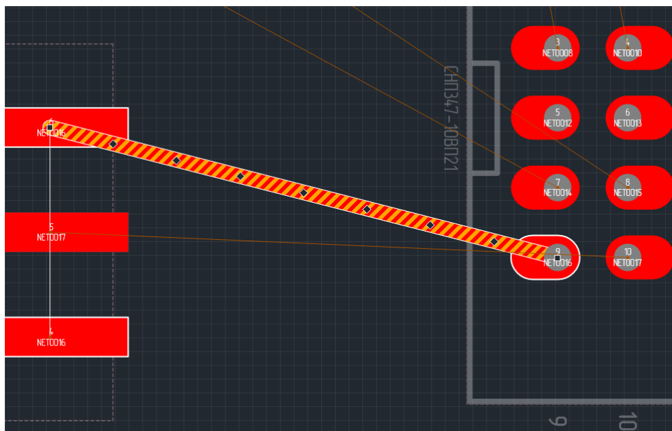
Рис. 269 Результат спрямления трека
