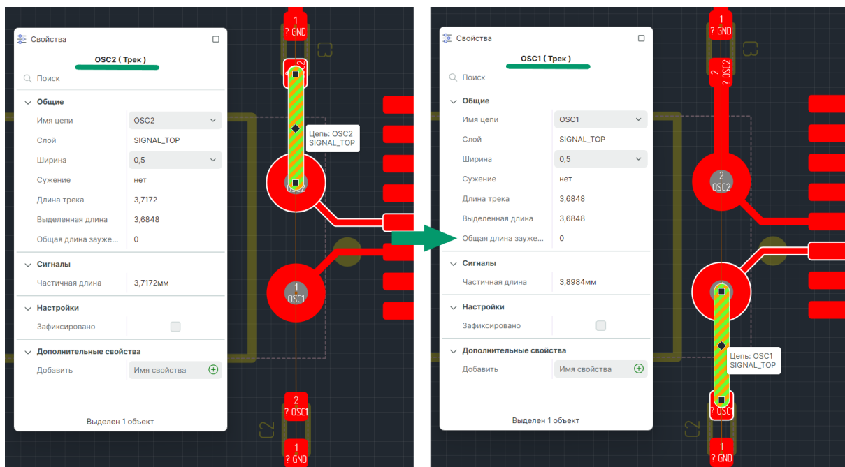
Рис. 422 Изменение цепи копии объекта при вставке с наложением на другой элемент печатного монтажа
