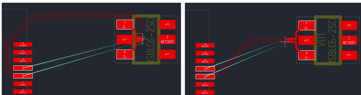
Рис. 332 Варианты соединения диффпары со стартовой парой контактных площадок
