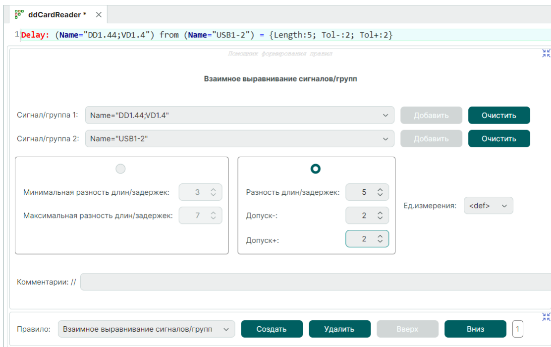
Рис. 371 Выравнивание длин/задержек сигналов внутри группы
