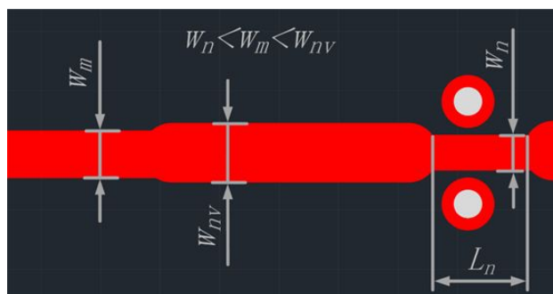
Рис. 202 Предопределенные значения трека
