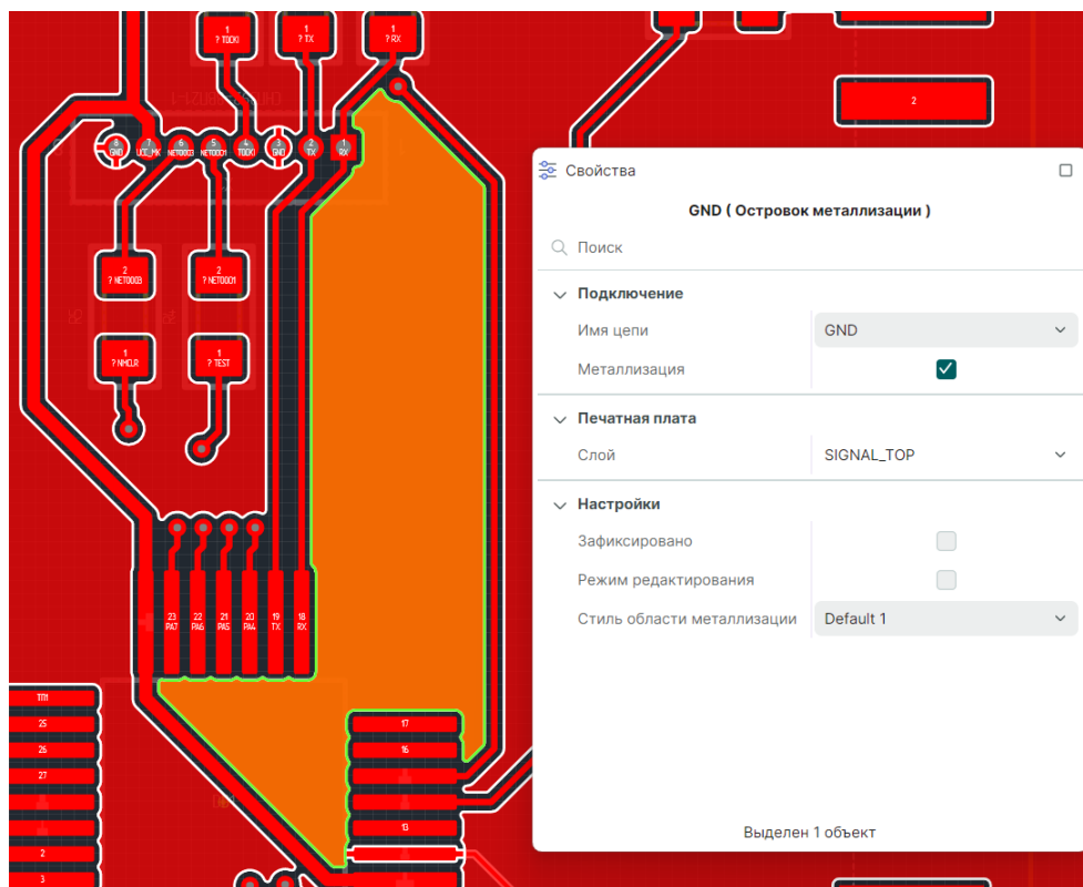
Рис. 460 Выделение островка области металлизации
