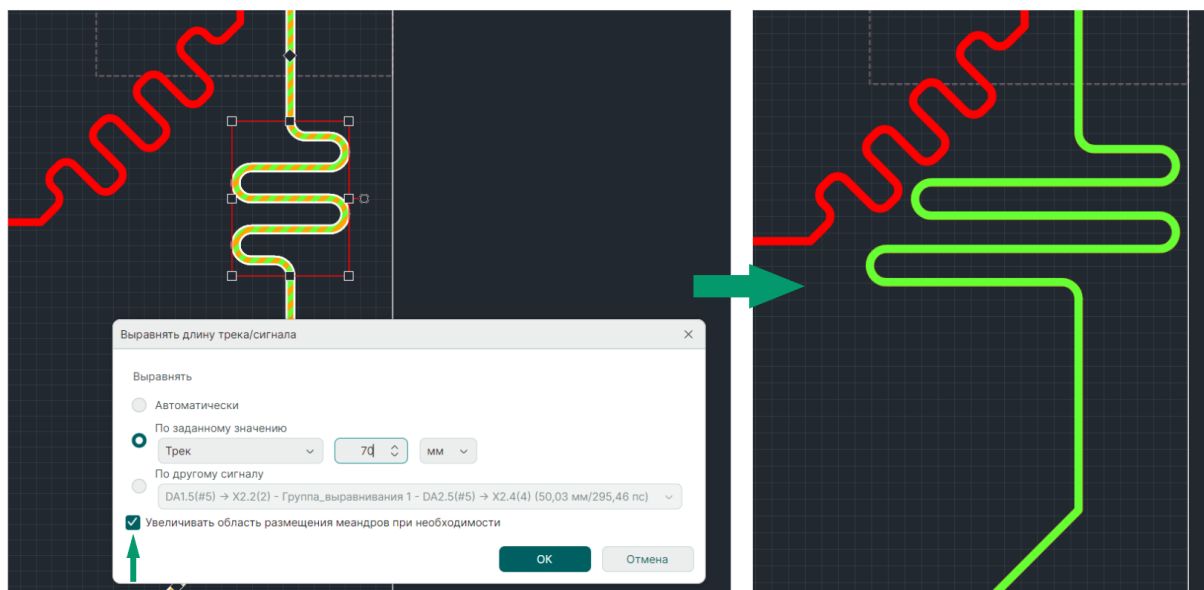
Рис. 393 Увеличение области размещения меандра
