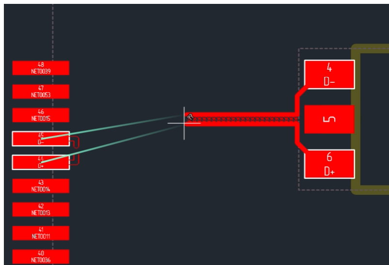
Рис. 335 Возможный вид прокладываемого участка диффпары
