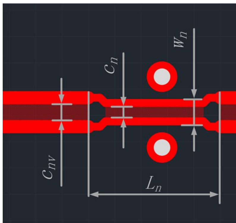
Рис. 325 Параметры диффпар
