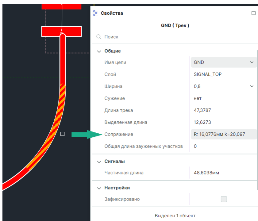
Рис. 283 Отображение свойств примененного скругления вершины трека
