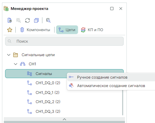
Рис. 360 Создание сигнала для выбранной сигнальной цепи в ручном режиме
