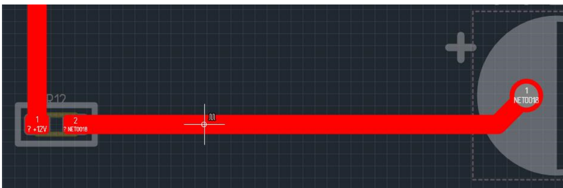
Рис. 270 Точка начала меандра
