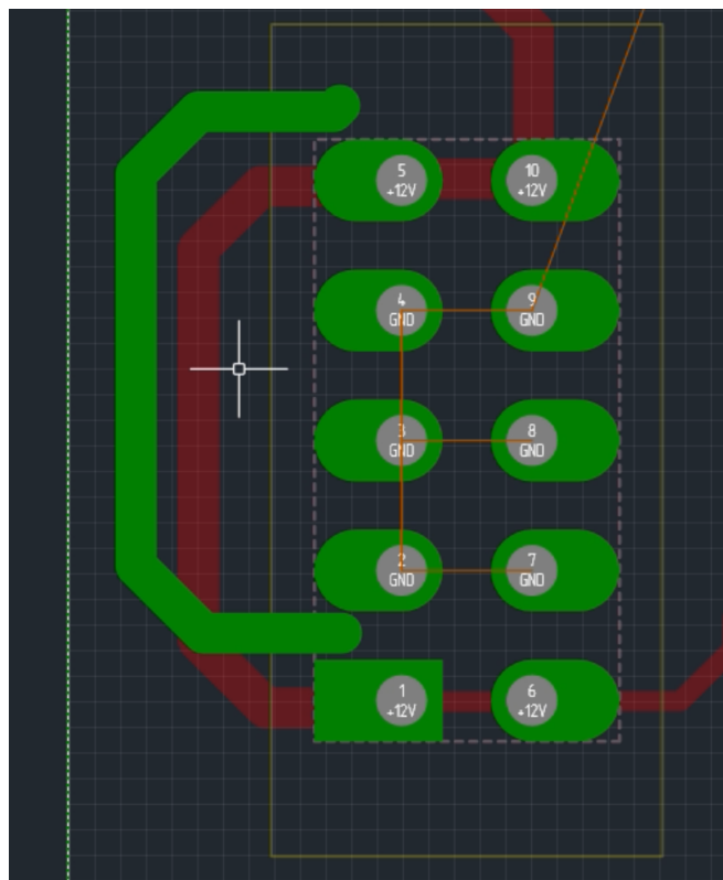
Рис. 419 Размещение скопированного трека
