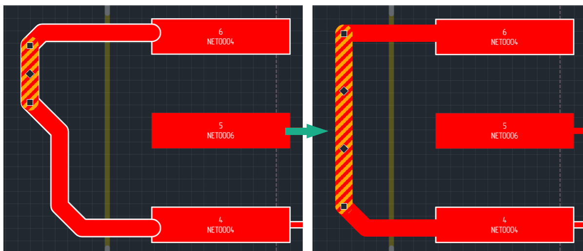
Рис. 260 Объединение сегментов трека
