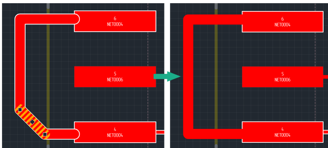
Рис. 259 Уменьшение количества сегментов трека
