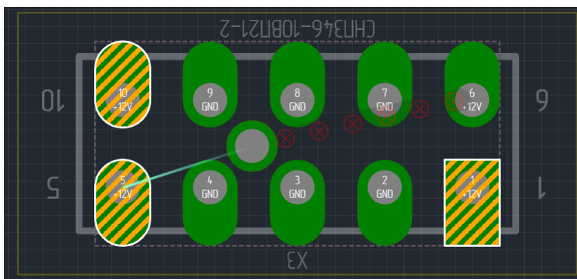
Рис. 222 Место, запрещенное для размещения перехода
