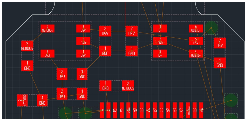
Рис. 196 Линии соединения
