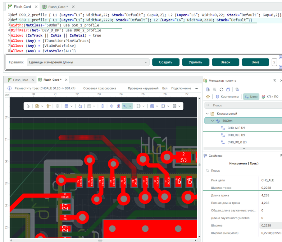
Рис. 53 Пример применения рассчитанных параметров к одиночной линии передачи в составе класса цепей
