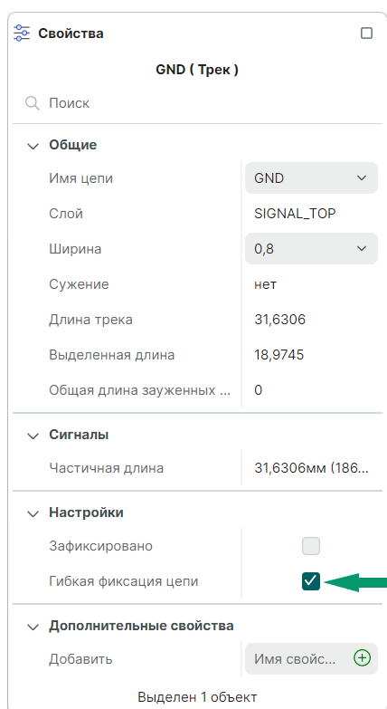
Рис. 91 Гибкая фиксация трека
