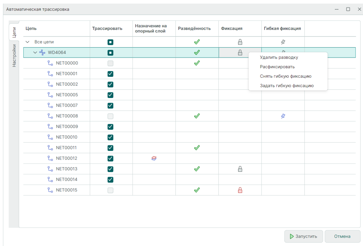
Рис. 398 Управление состоянием трассировки и фиксации
