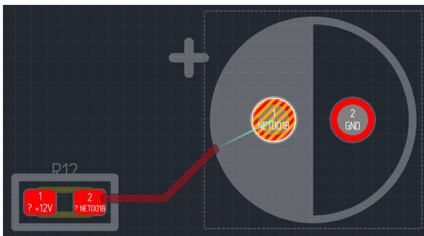
Рис. 211 Измененная комбинация отрезков при соединении двух точек треком
