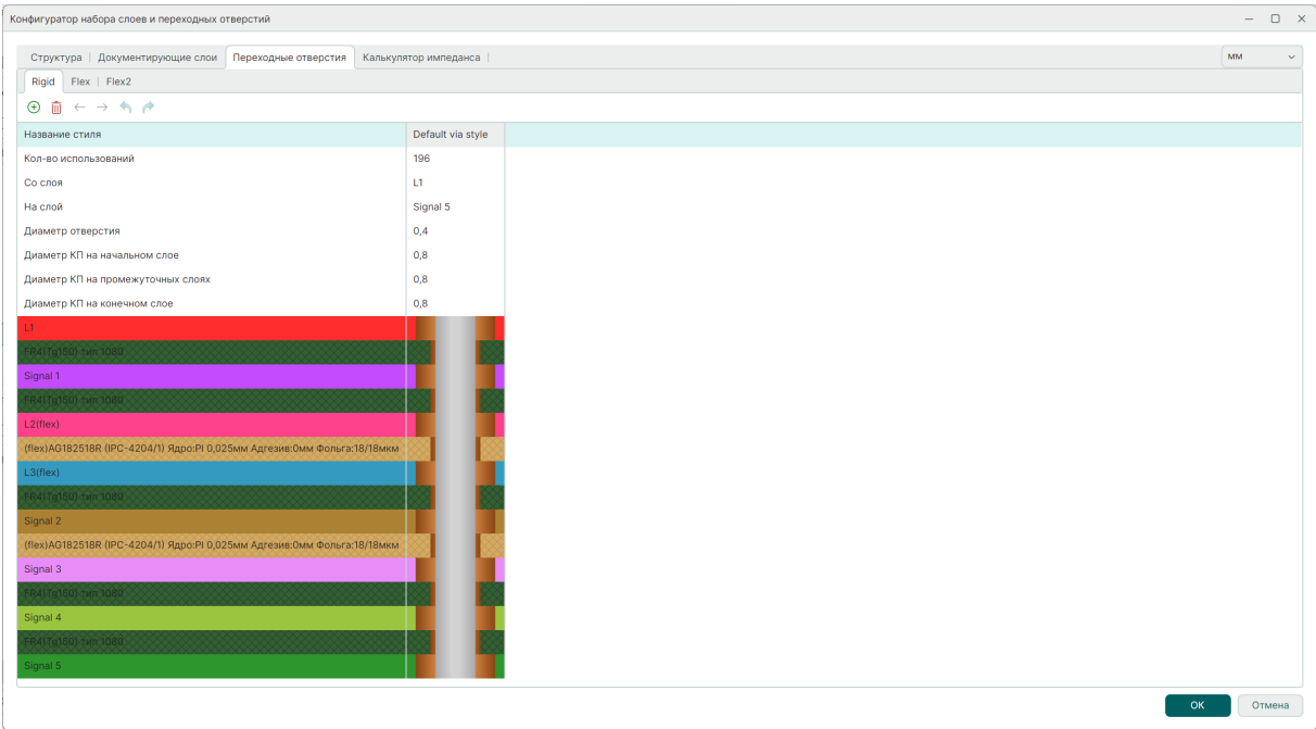
Рис. 34 Окно редактора слоев. Вкладка «Переходные отверстия»
