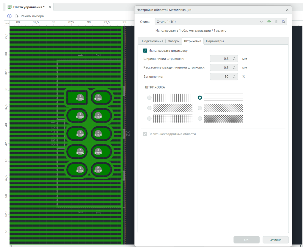
Рис. 452 Пример горизонтального штрихового заполнения области металлизации
