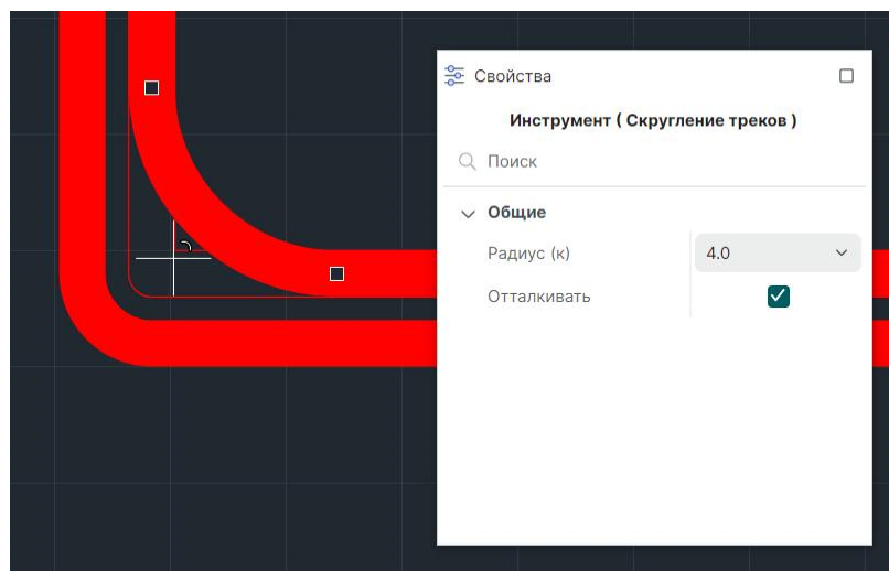
Рис. 347 Скругление угла на "расстегнутом" участке диффпары
