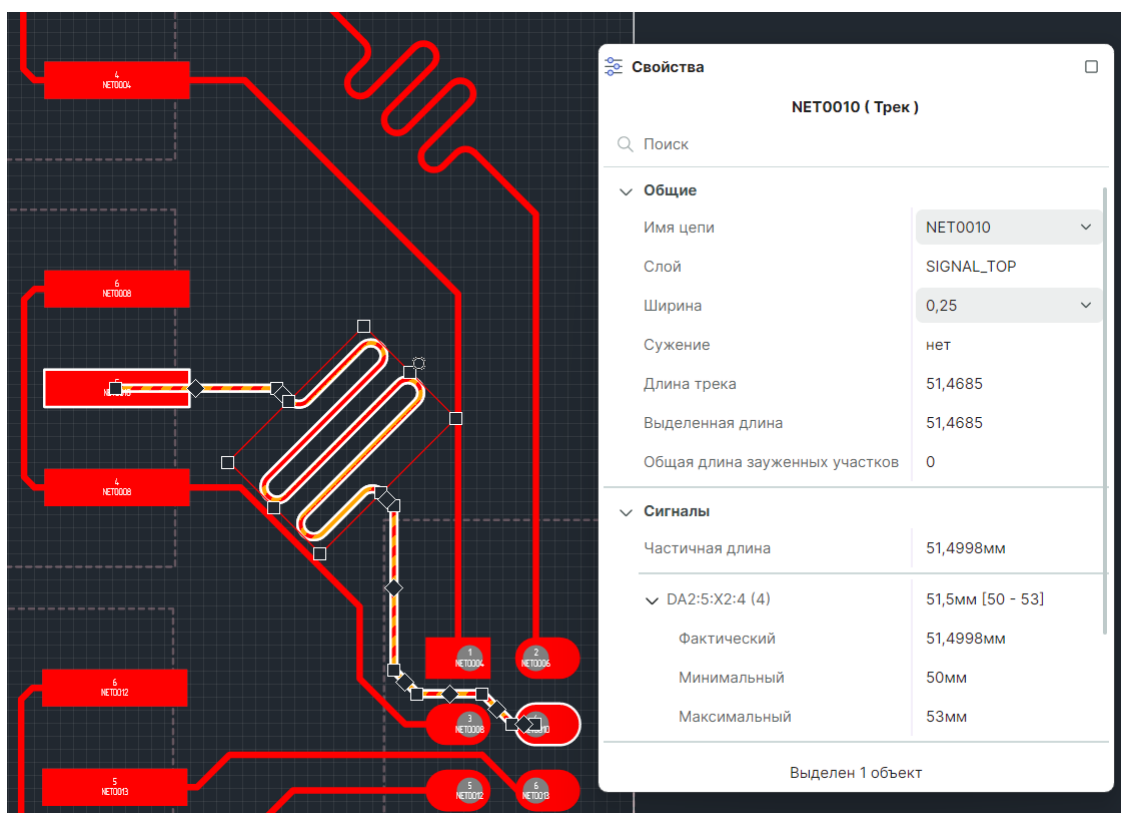
Рис. 387 Выравнивание длины сигнала в режиме «Автоматически»
