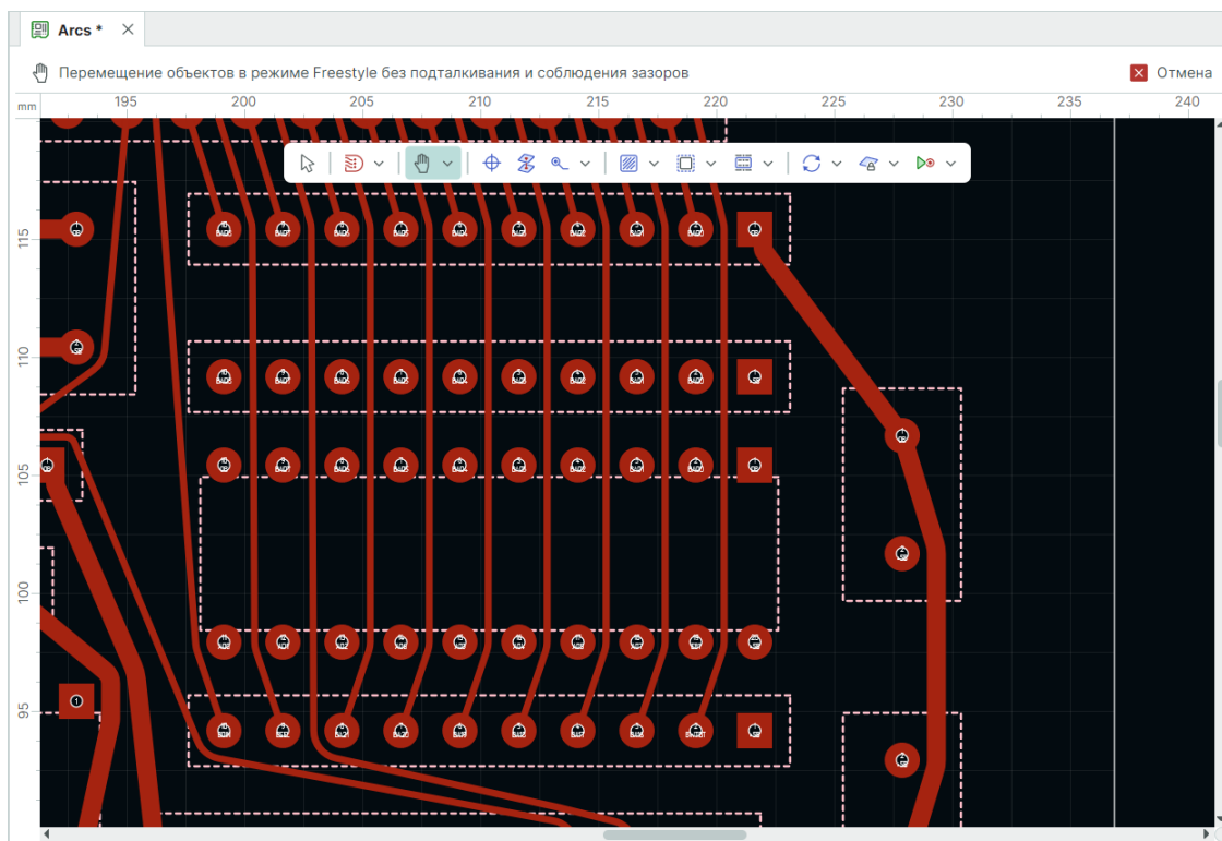
Рис. 409 Перемещение проводников в режиме Freestyle
