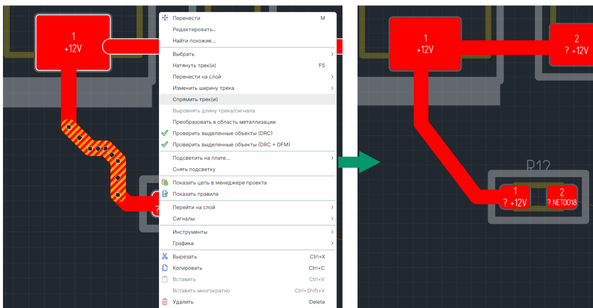
Рис. 216 Спрямление участка трека
