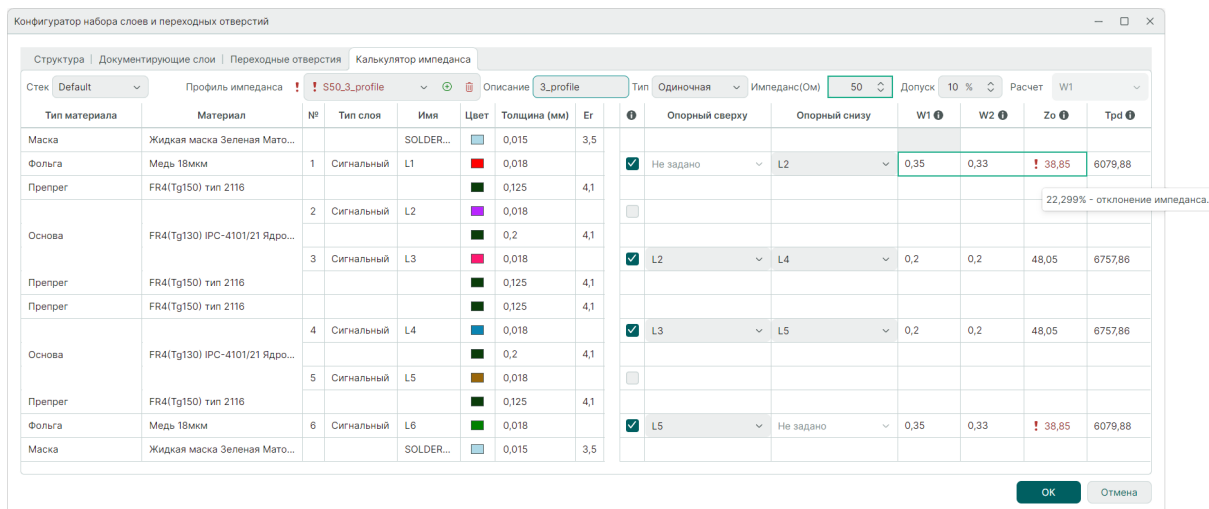
Рис. 47 Профиль импеданса с заданными значениями волнового сопротивления и ширины проводника
