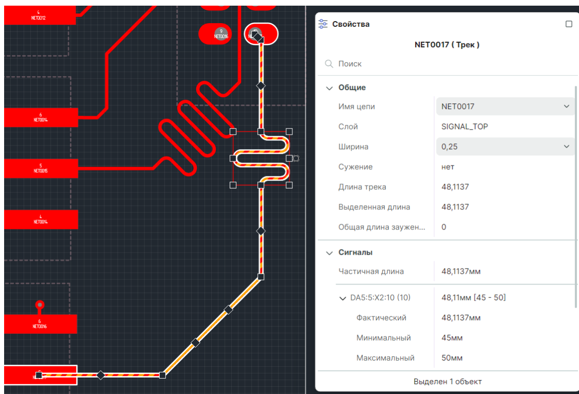
Рис. 390 Выравнивание длины сигнала в режиме «По другому сигналу»
