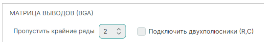
Рис. 308 Исключение внешних рядов и колонок из матрицы BGA при построении фанатов
