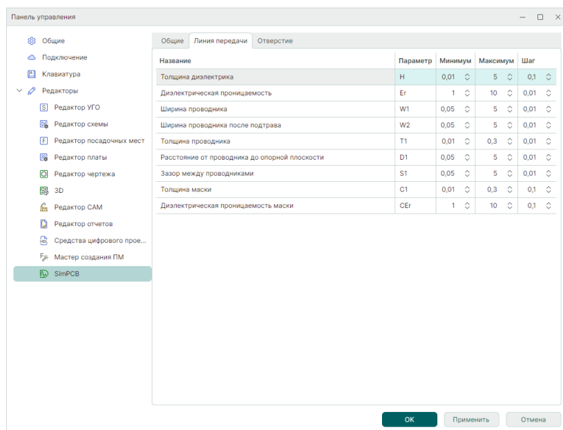
Рис. 142 Параметры линии передачи
