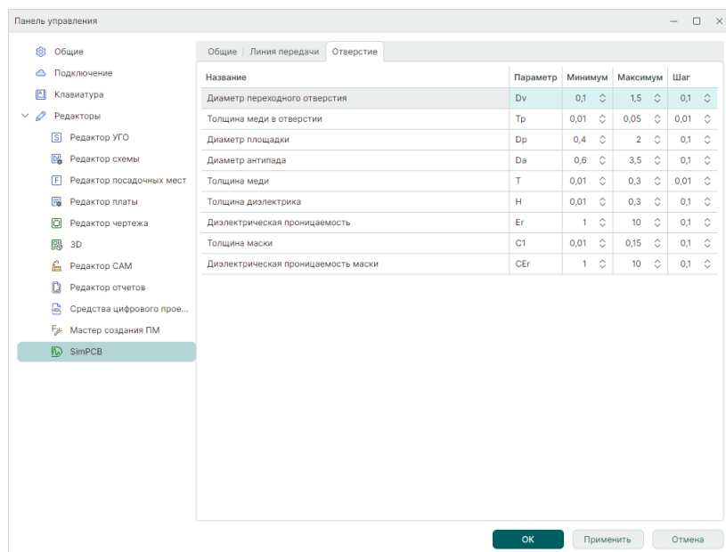
Рис. 143 Параметры отверстия
