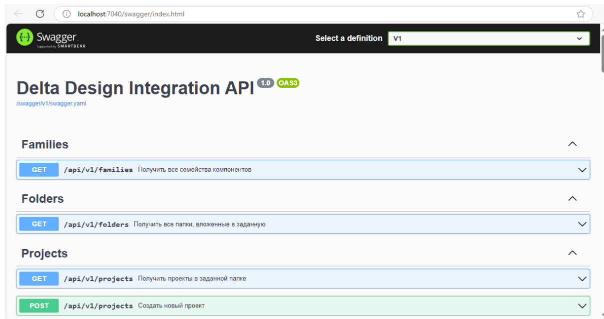
Рис. 143 Описание программного интерфейса
