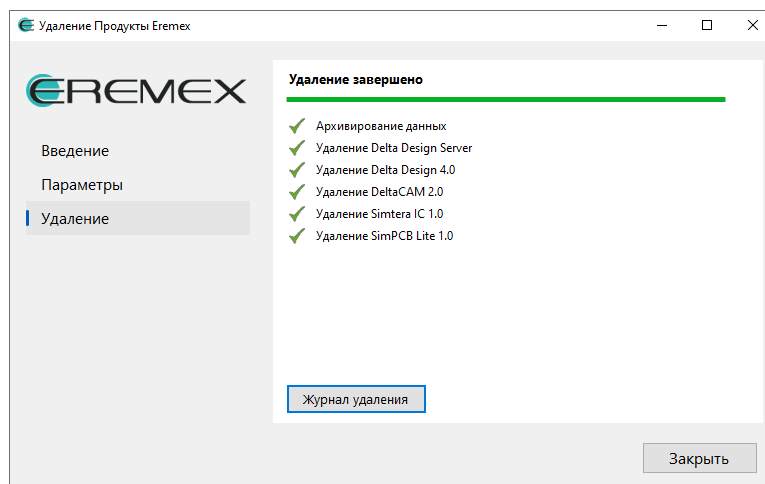
Рис. 63 Завершение удаления
