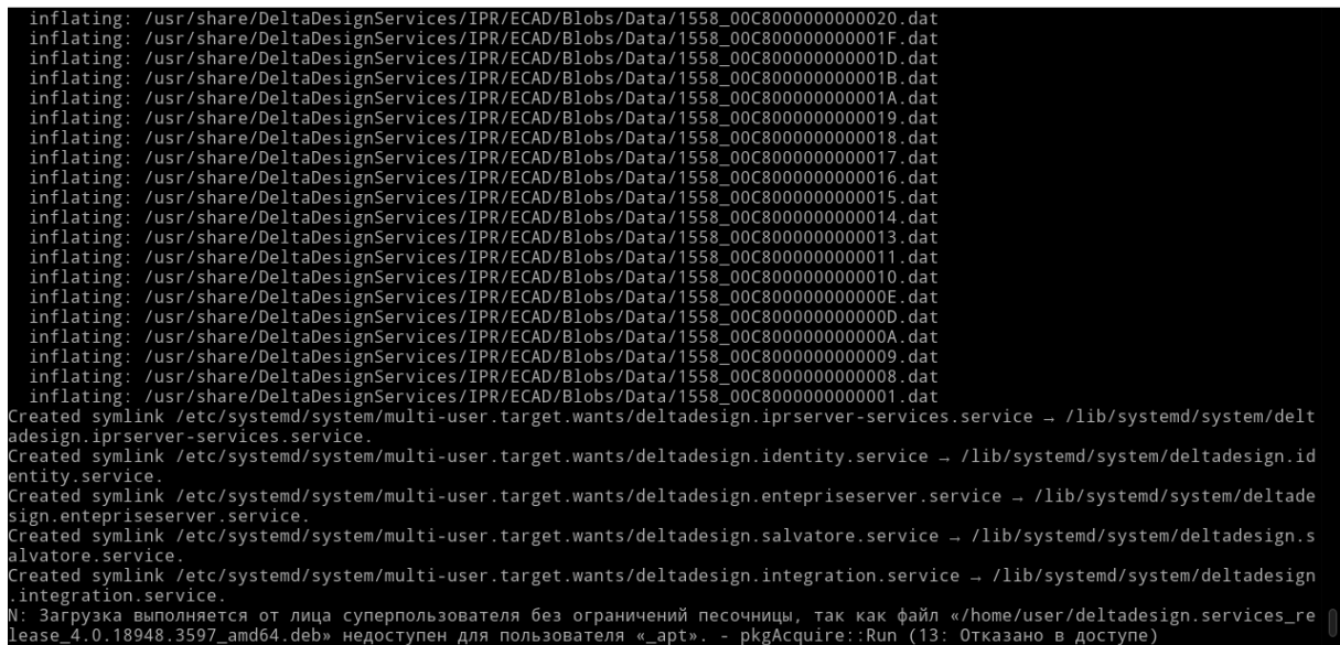
Рис. 60 Завершение установки
