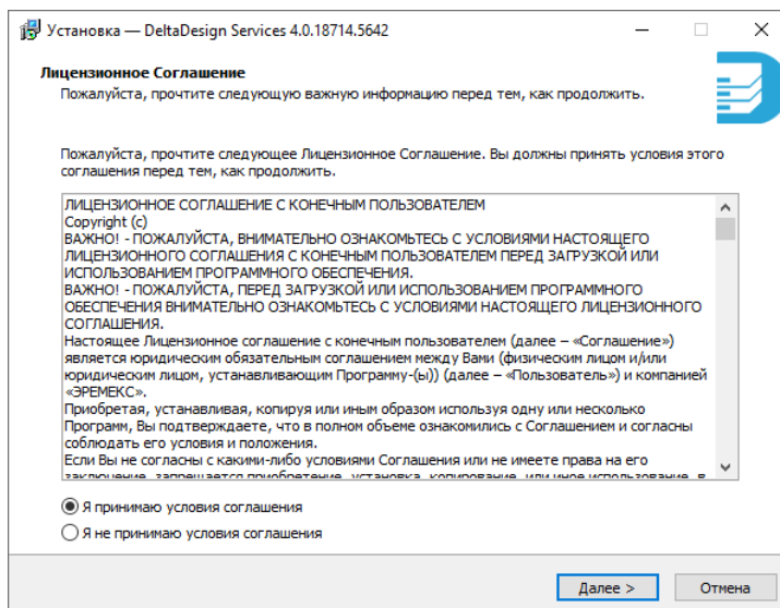
Рис. 22 Лицензионное соглашение
