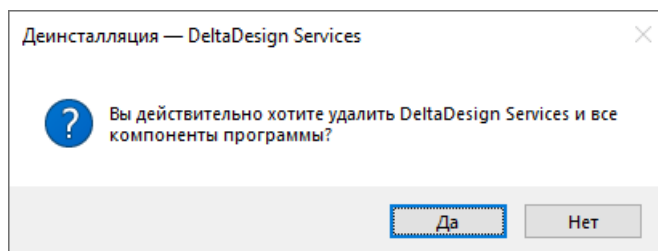
Рис. 64 Подтверждение удаления
