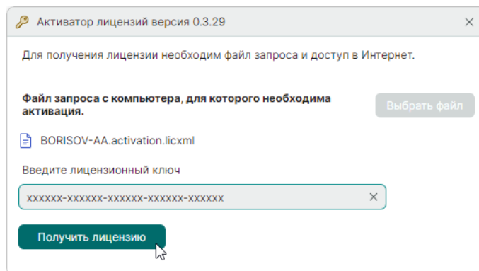
Рис. 73 Получение лицензии
