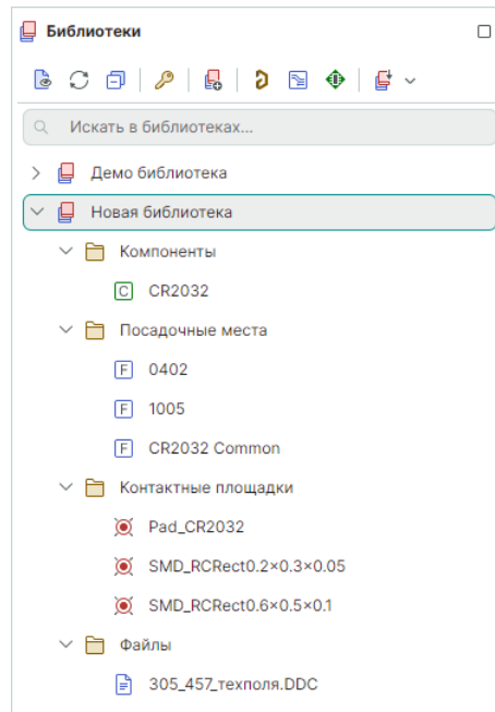
Рис. 125 Панель «Библиотеки»
