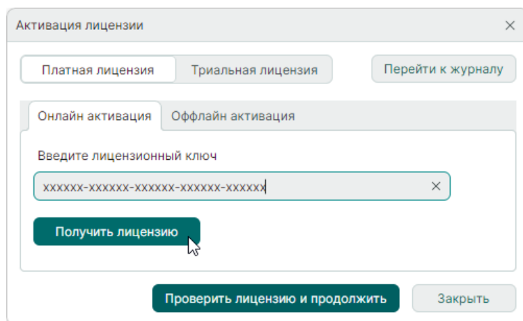
Рис. 67 Получение лицензии
