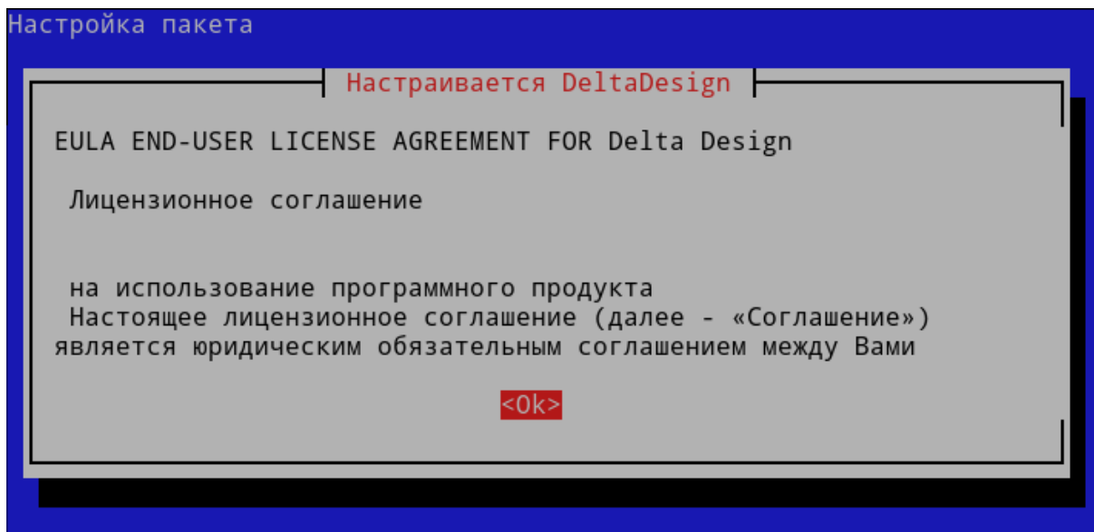
Рис. 45 Лицензионное соглашение
