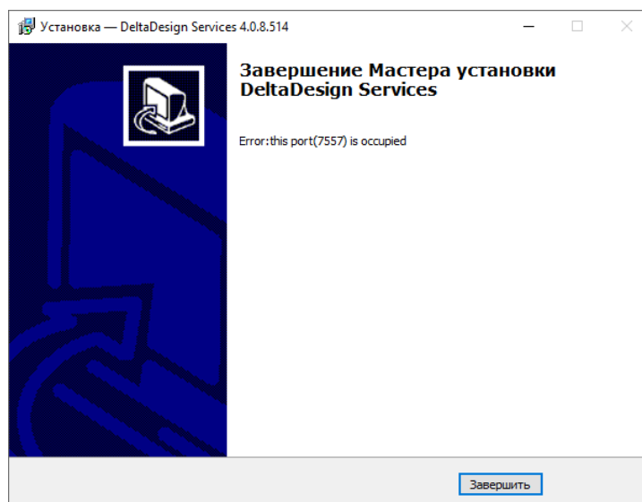
Рис. 39 Завершение установки
