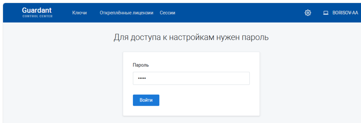
Рис. 97 Ввод пароля
