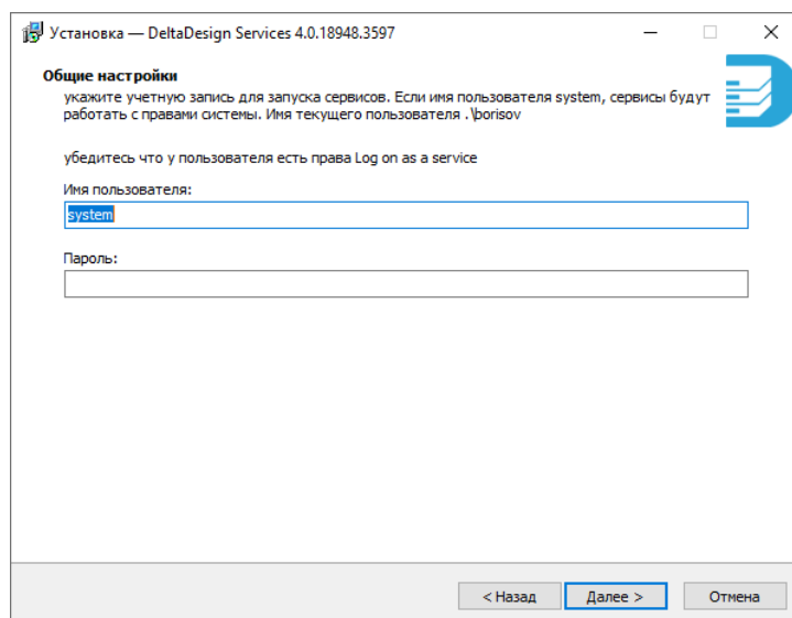
Рис. 25 Общие настройки
