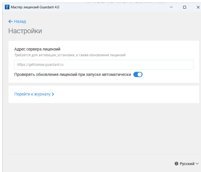
Рис. 90 Адрес сервера лицензий
