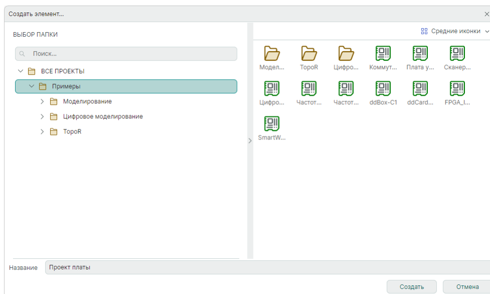
Рис. 13 Выбор папки
