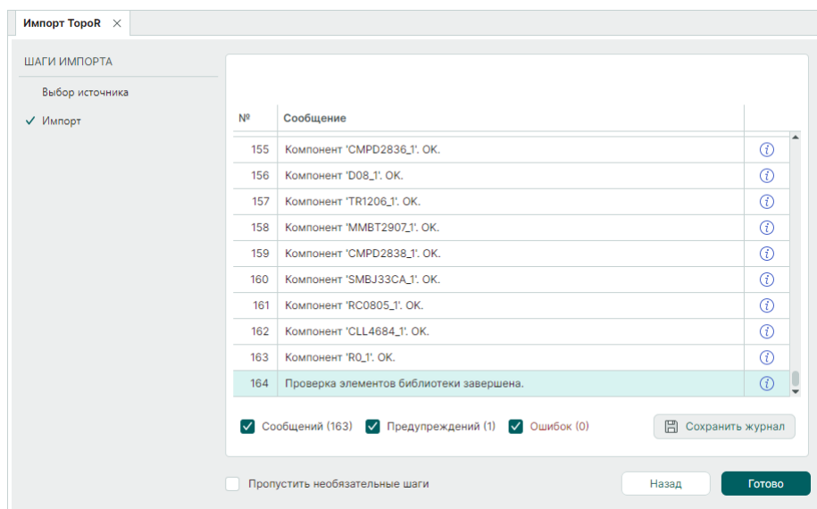
Рис. 68 Завершение импорта
