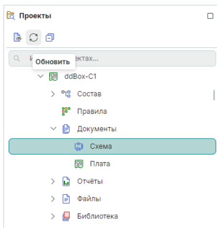
Рис. 9 Обновить дерево
