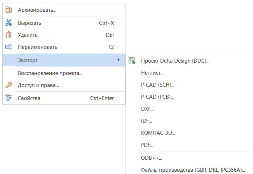
Рис. 69 Экспорт проекта
