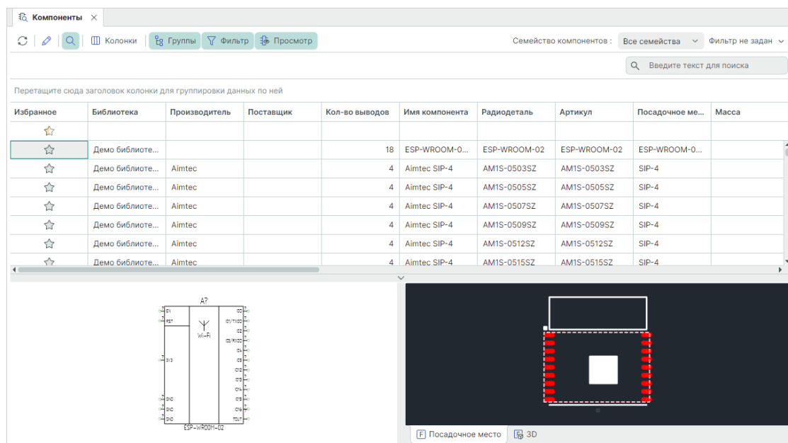
Рис. 45 Окно «Компоненты»
