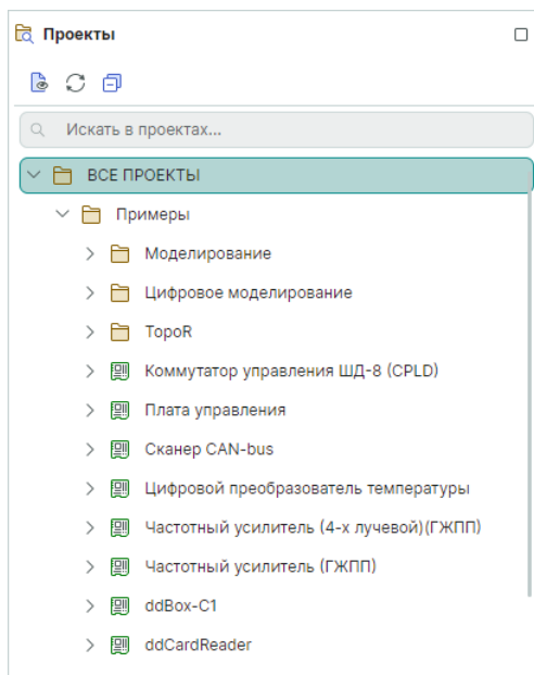
Рис. 3 Дерево проектов
