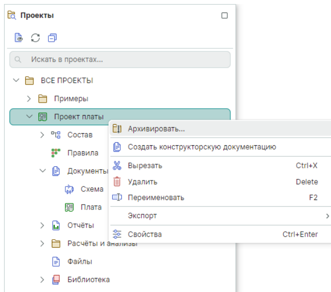
Рис. 40 Архивирование проекта
