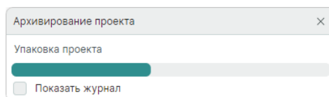
Рис. 41 Процесс архивации
