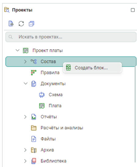
Рис. 27 Создание блока
