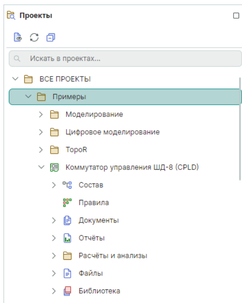
Рис. 1 Панель «Проекты»
