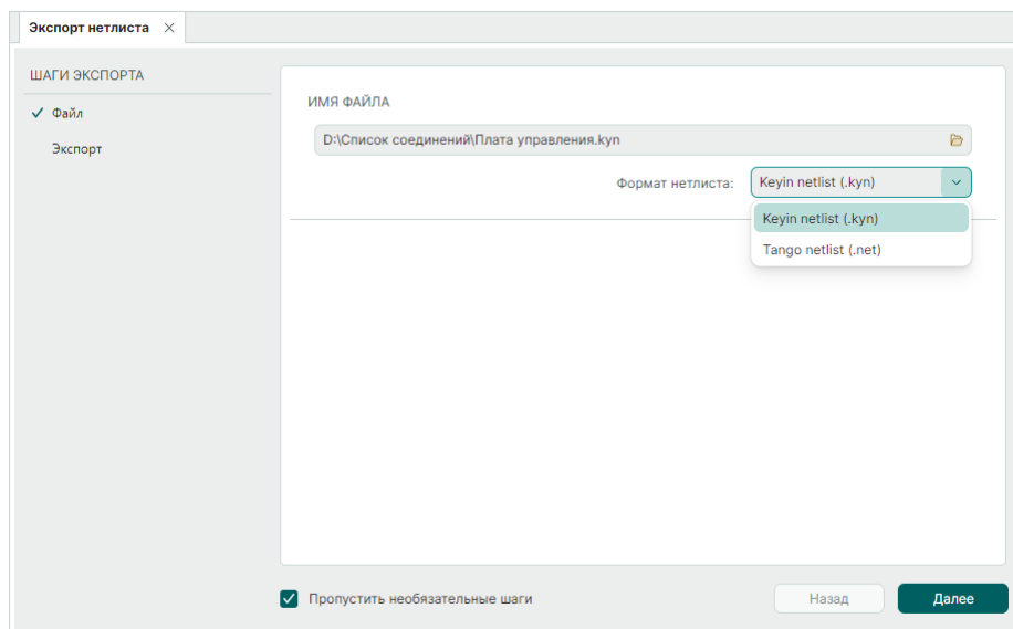
Рис. 78 Выбор формата
