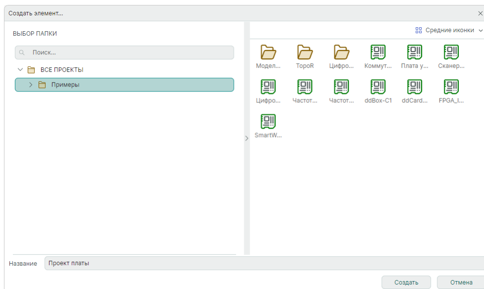
Рис. 22 Выбор папки
