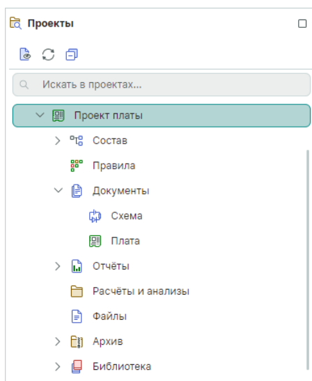
Рис. 26 Структура проекта
