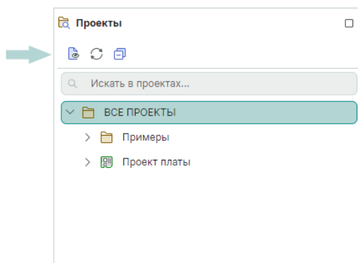
Рис. 6 Панель инструментов
