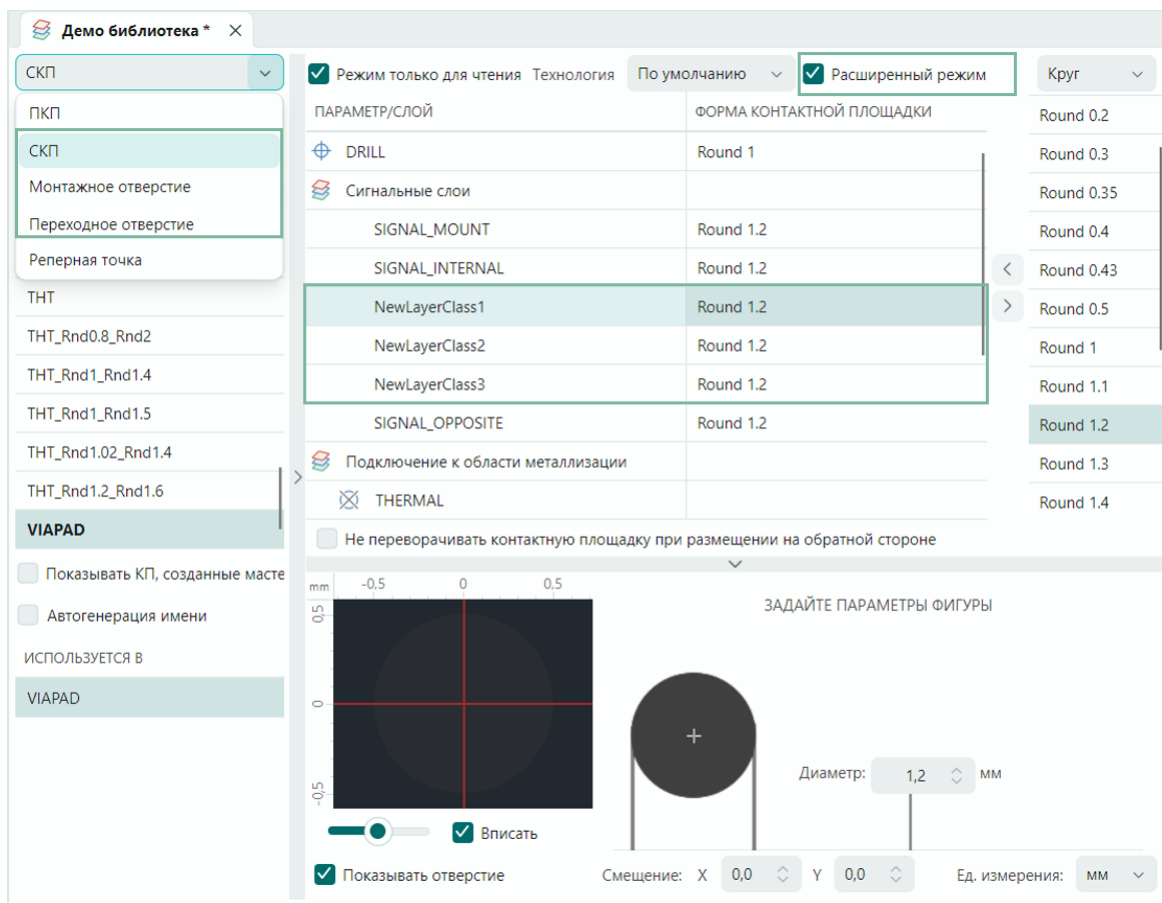
Рис. 101 Редактор контактных площадок
