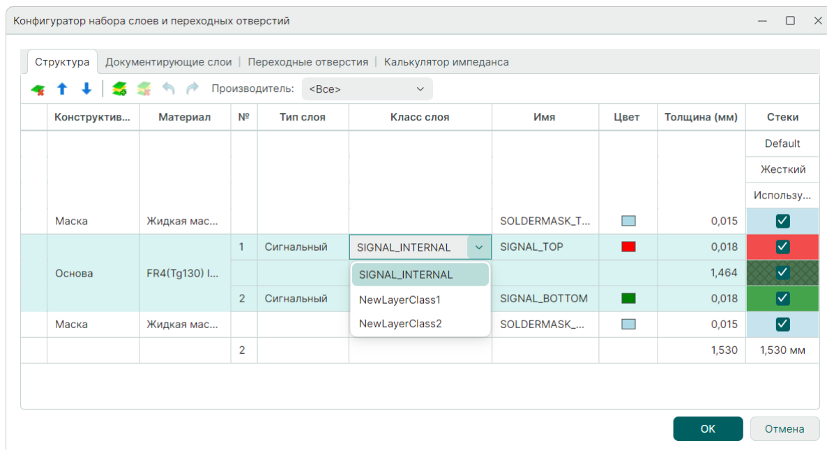
Рис. 99 Выбор внутреннего сигнального класса слоев
