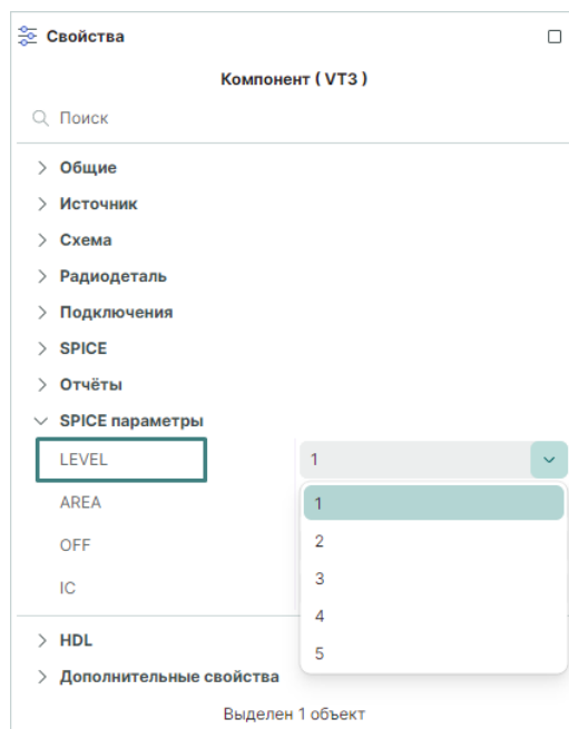
Рис. 51 Редактируемые SPICE-параметры
