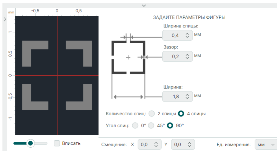
Рис. 65 Задание параметров термобарьера
