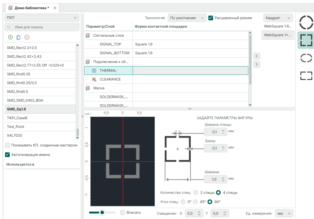
Рис. 63 Выбор параметра «THERMAL» для установки термобарьера
