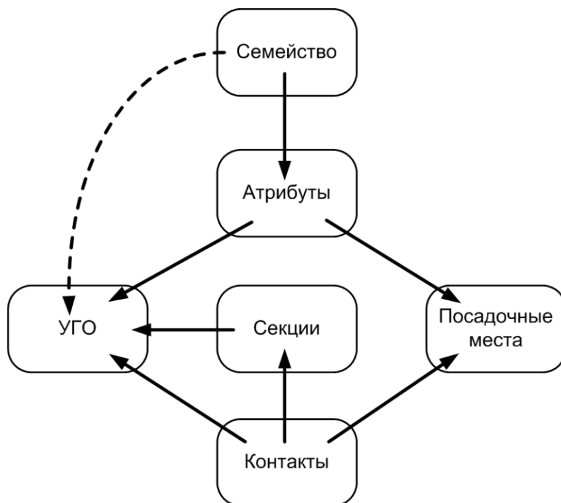
Рис. 1 Структурная схема описания компонента в Delta Design
