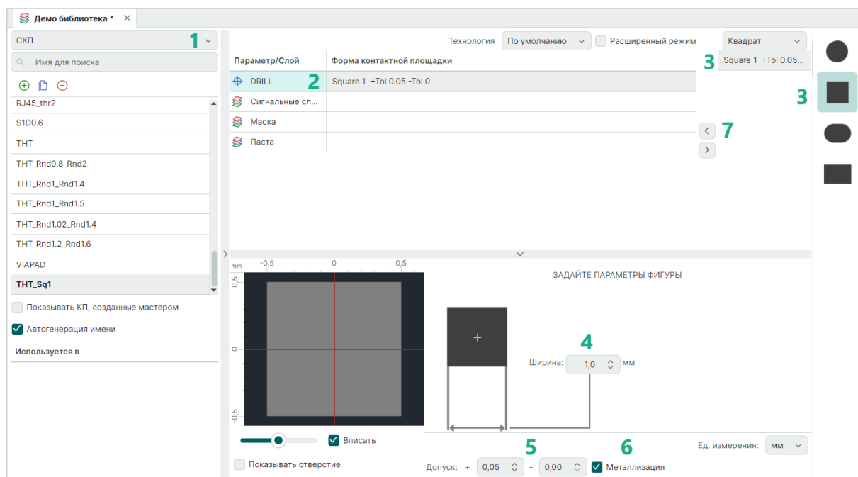
Рис. 56 Создание отверстия для контактной площадки
