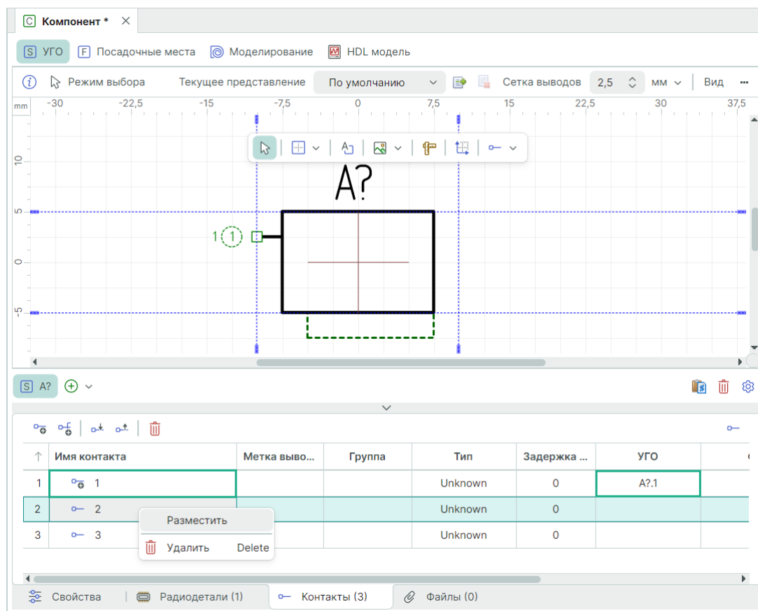
Рис. 237 Размещение выводов на основе контактов
