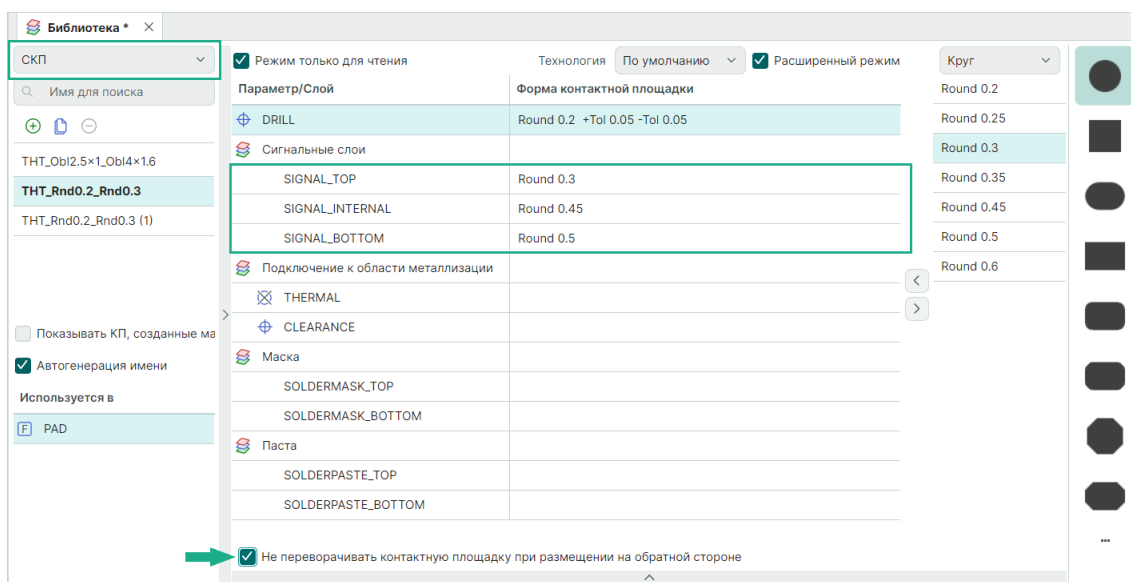
Рис. 59 Функция «Не переворачивать контактную площадку при размещении на обратной стороне»
