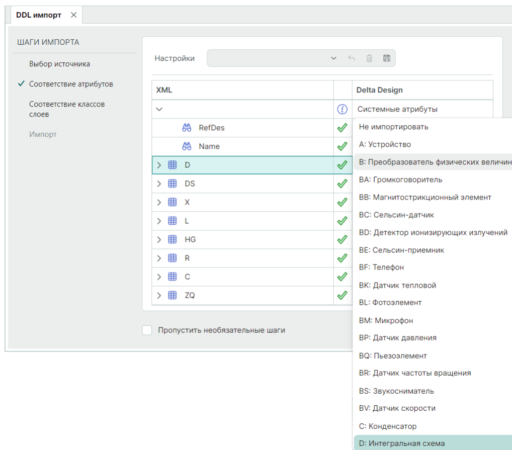
Рис. 24 Сопоставление атрибутов при импорте
