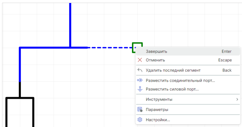
Рис. 64 Завершение работы инструмента «Разместить проводник»
