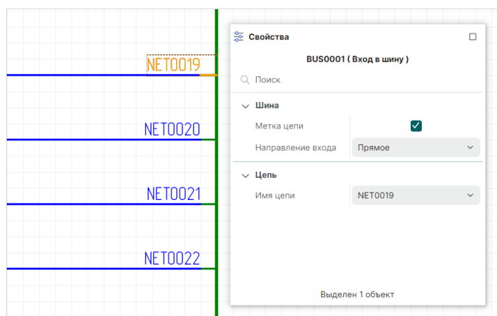
Рис. 168 Подключение цепи к шине (Вход в шину)
