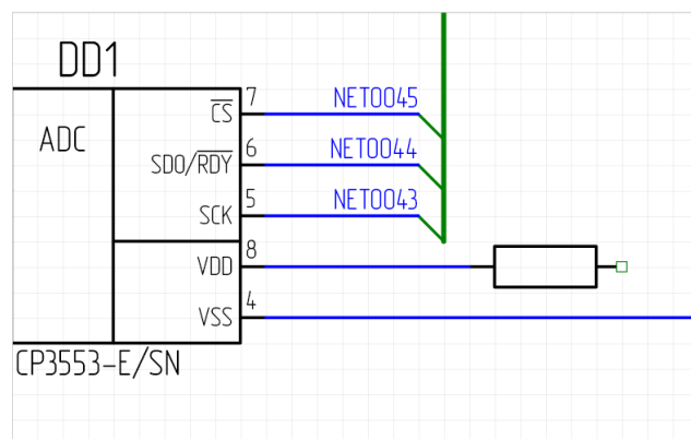
Рис. 69 Пример выполнения команды «Подключить вывод(ы)»
