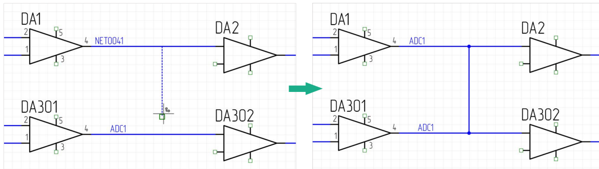
Рис. 136 Изменение имен при соединении цепей
