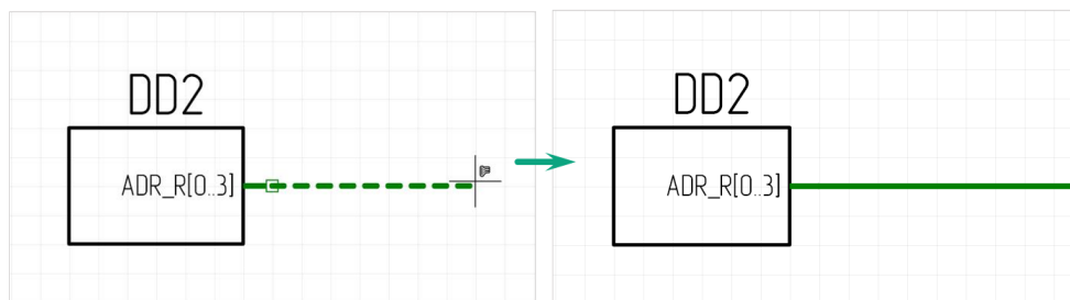
Рис. 194 Подключение шины к групповому выводу
