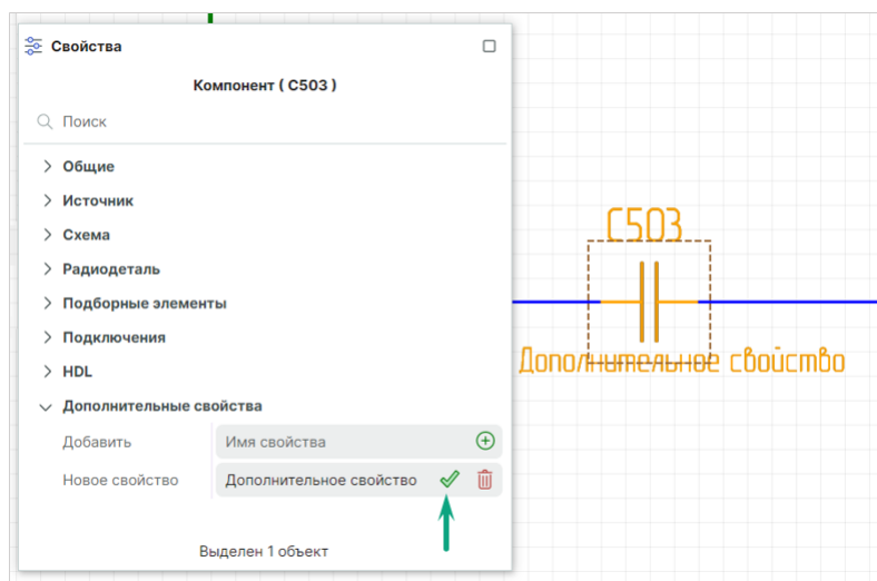
Рис. 107 Отображение значения дополнительного атрибута на УГО
