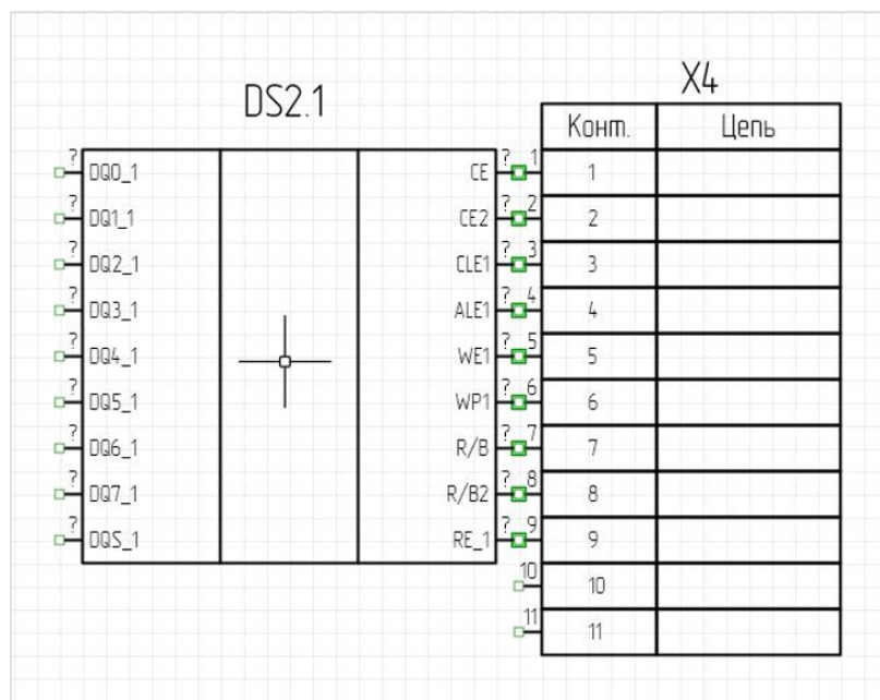
Рис. 163 Размещение радиодетали на выводы УГО другой радиодетали
