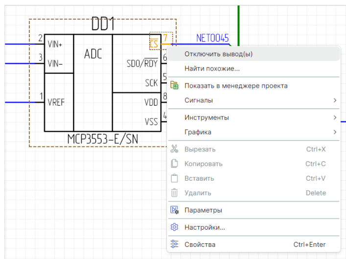
Рис. 70 Контекстное меню подключенного вывода
