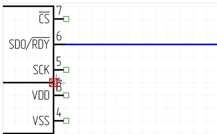
Рис. 61 Точка, недоступная для размещения проводника
