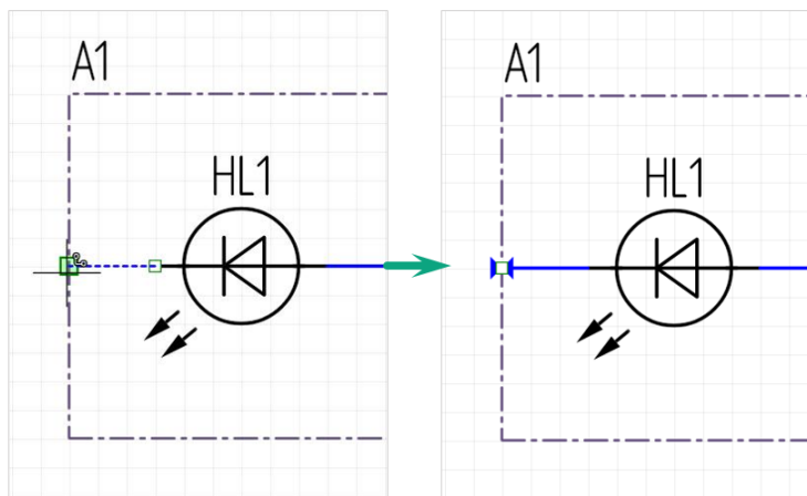
Рис. 258 Завершение цепи на границе блока
