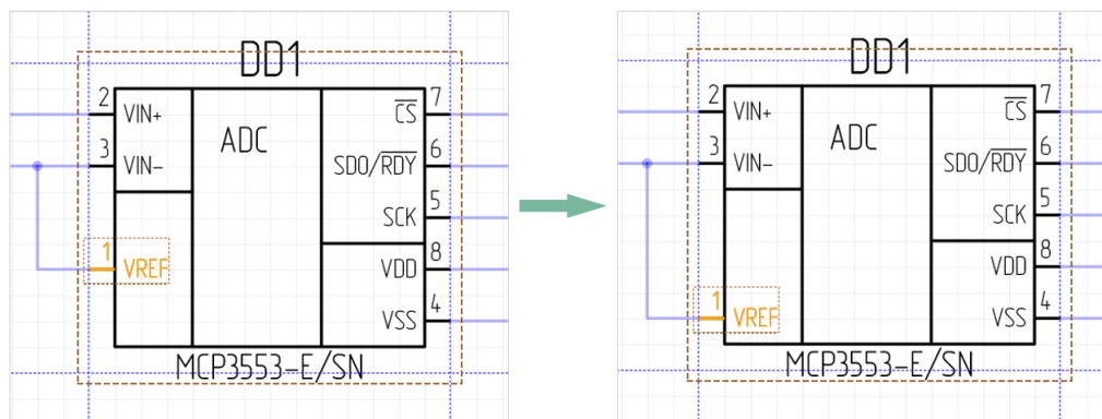
Рис. 39 Перемещение выводов УГО на схеме
