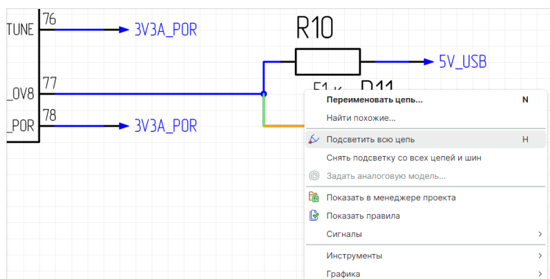
Рис. 155 Вызов функции «Подсветить всю цепь»
