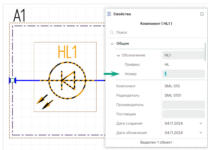
Рис. 263 Корректировка нумерации компонента встроенного блока
