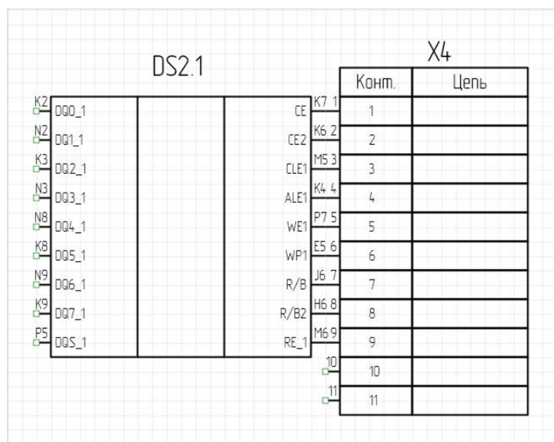
Рис. 164 Радиодеталь, размещенная на выводах УГО другой радиодетали
