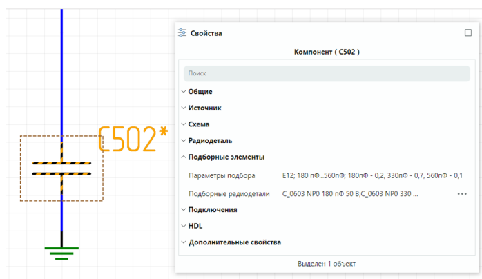
Рис. 92 Позиционное обозначение компонента с подборными элементами
