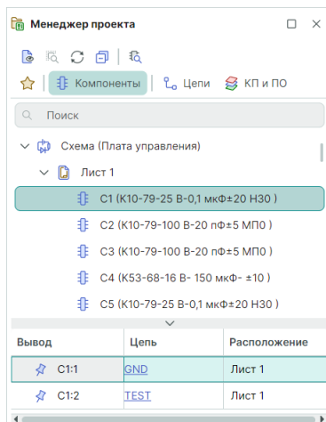
Рис. 227 Подробная информация о выводах УГО
