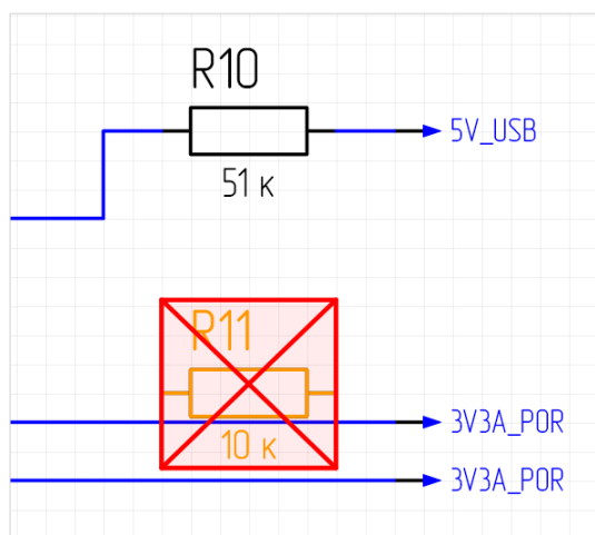
Рис. 158 УГО в области, недоступной для размещения
