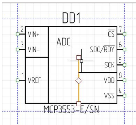
Рис. 38 Произвольное изменение графических объектов редактируемого УГО
