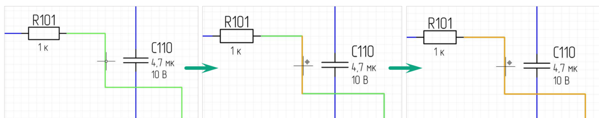
Рис. 75 Выбор сегмента проводника и проводника целиком
