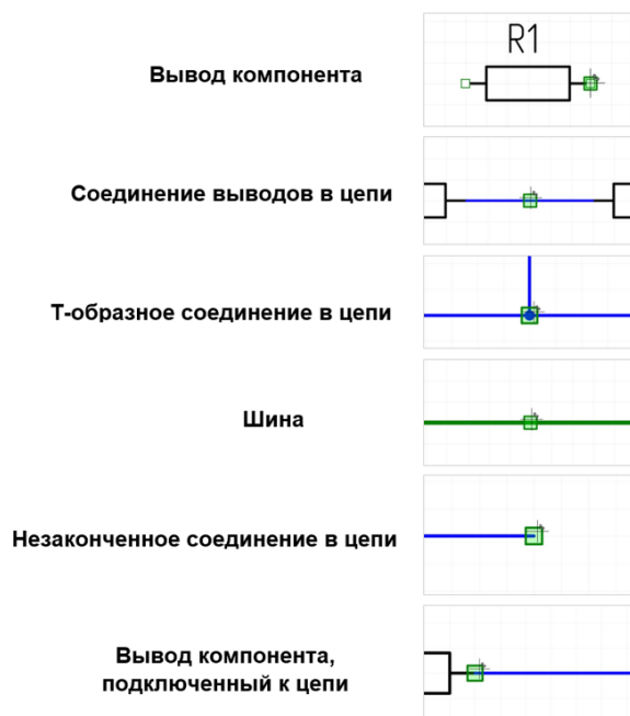
Рис. 55 Список разрешенных и запрещенных объектов для начальных и конечных точек соединений на электрической схеме
