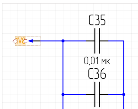
Рис. 205 Начало выбора объектов (старт - метка порта)
