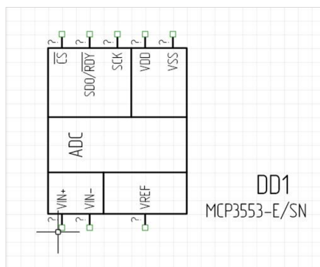
Рис. 32 Поворот УГО при размещении радиодетали на схеме
