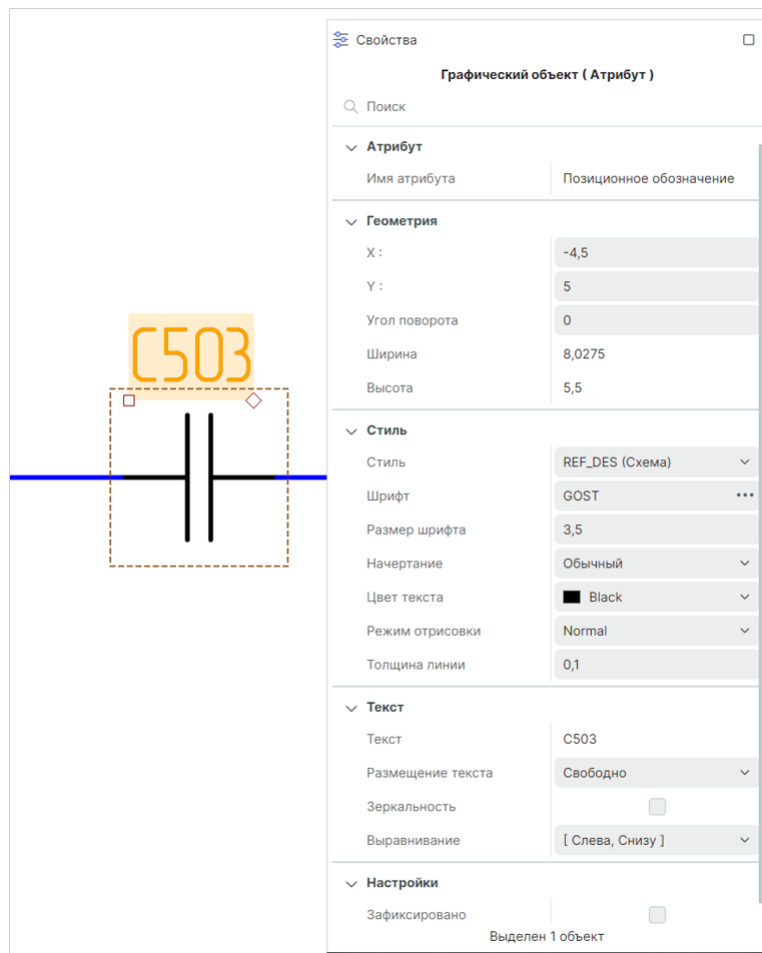
Рис. 110 Свойства позиционного обозначения
