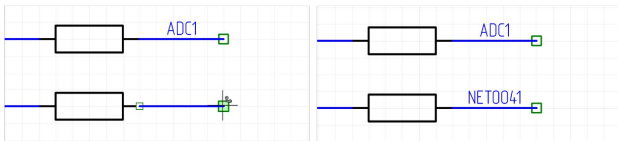
Рис. 126 Незавершенная цепь
